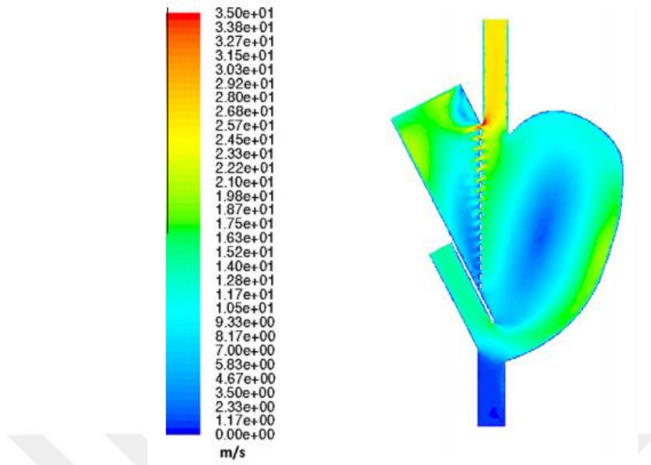
Şekil 6.1 Ayrım bölgesi etrafındaki akış hızları [40]
