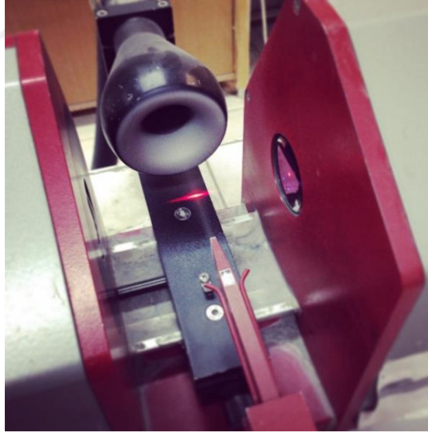
Şekil 7.1 Lazer kırınımı ile tane boyu dağılımı belirleme cihazı
