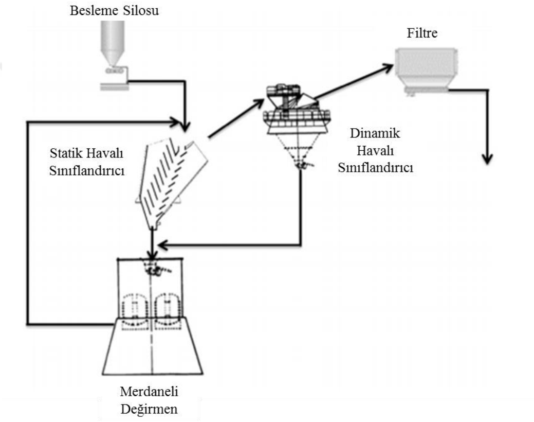
Şekil 3.2 Dik değirmende öğütme akım şeması [24]
