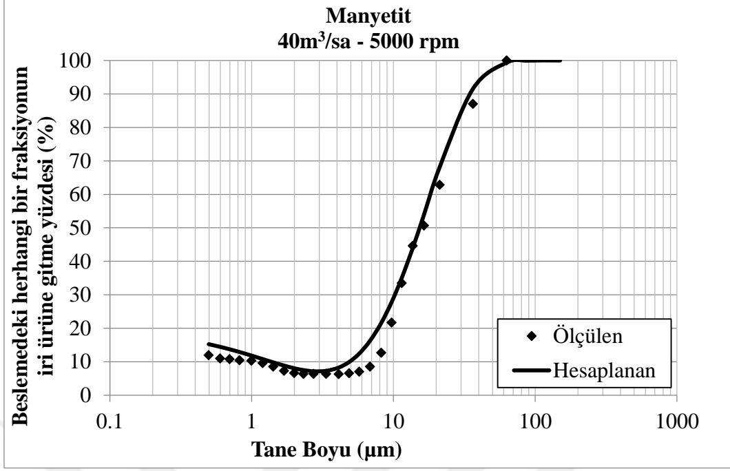
Şekil 7.32 Manyetit için 40 m 3 /sa - 5000 rpm koşullarında ölçülen ve hesaplanan verimlilik eğrileri
