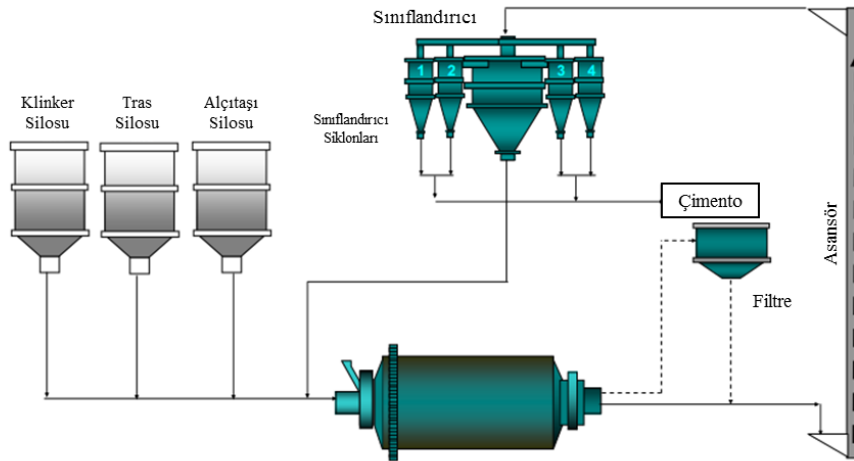
Şekil 3.4 Kapalı devre akım şeması [28]
