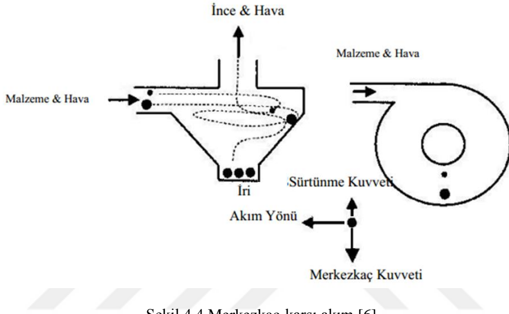
Şekil 4.4 Merkezkaç-karşı akım [6]
