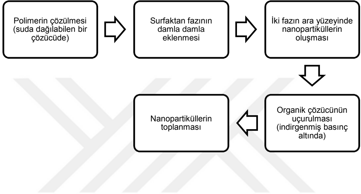
Şekil- 11: Nanoçöktürme metodunun basamakları 27
