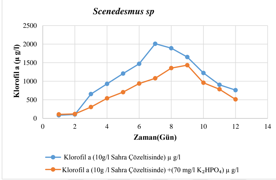
Şekil 4.48. 10g/l içeren Sahra çözeltisi ve bu çözeltiliye ilave edilen 70mg/l fosfat içeren çözeltilide Scenedesmus sp 'de ortalama klorofil a değişimi.
