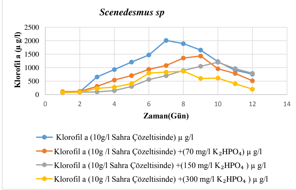
Şekil 4.47. Sahra çözeltili ve farklı fosfat içeren Sahra çözeltilerinde Scenedesmus sp 'de ortalama klorofil a değişimi
