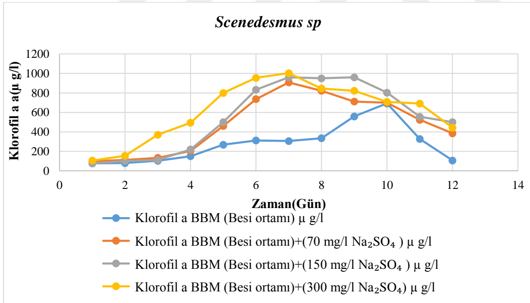
Şekil 4.41. BBM ortamında değişik Sülfat artışında Scenedesmus sp 'de ortalama klorofil a değişimi (µg/l)
