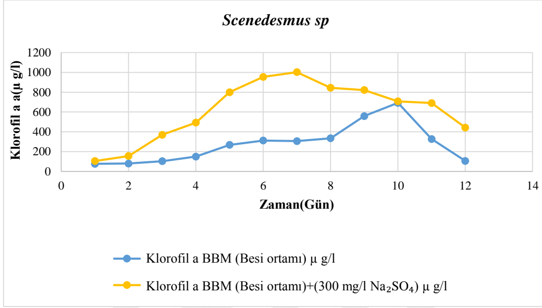
Şekil 4.42. BBM ortamında ve BBM ortamına 300 (mg/l) Na 2 SO 4 ilave edilen halde Scenedesmus sp 'de ortalama klorofil a değişimi(µg/l)
