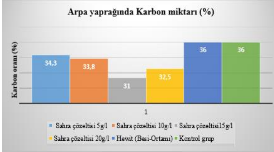
Şekil 4.62. Deęişik besi ortamlarında yetiştirilen arpa 'da 20 gün sonunda ölçülen ortalama karbon deęerleri (%)
