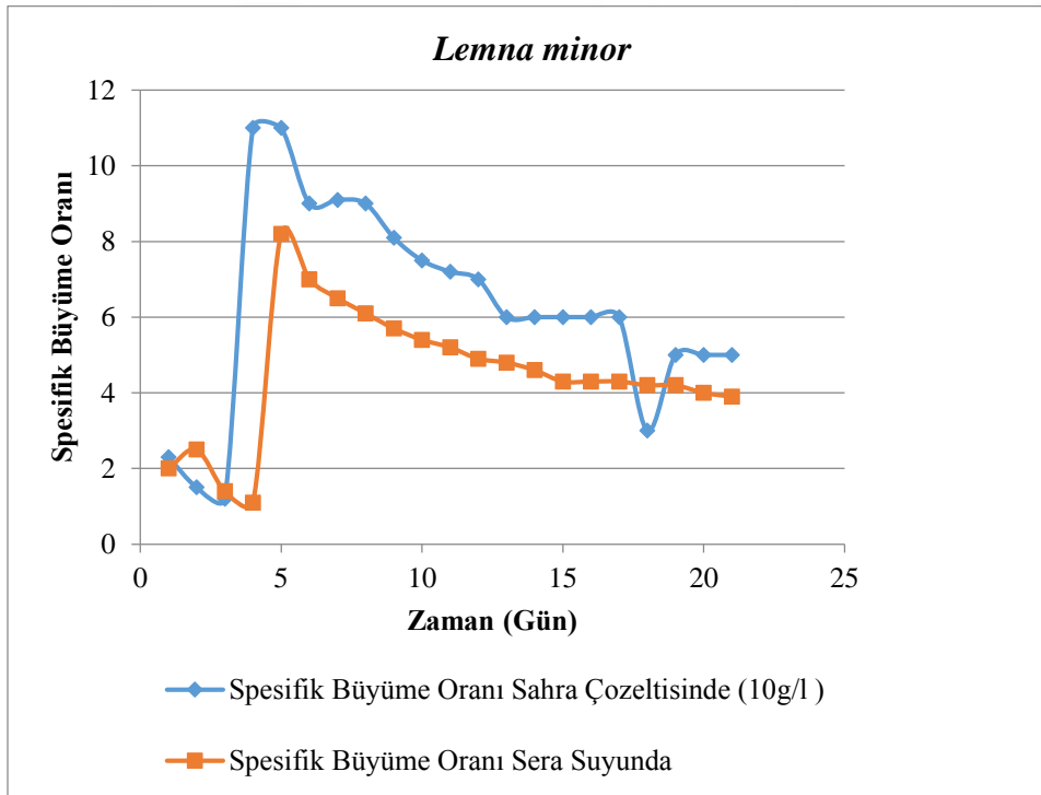
Şekil 4.49. Lemna minör ' de Sahra çözeltisinde ve sera suyunda spesifik büyüme oranı
