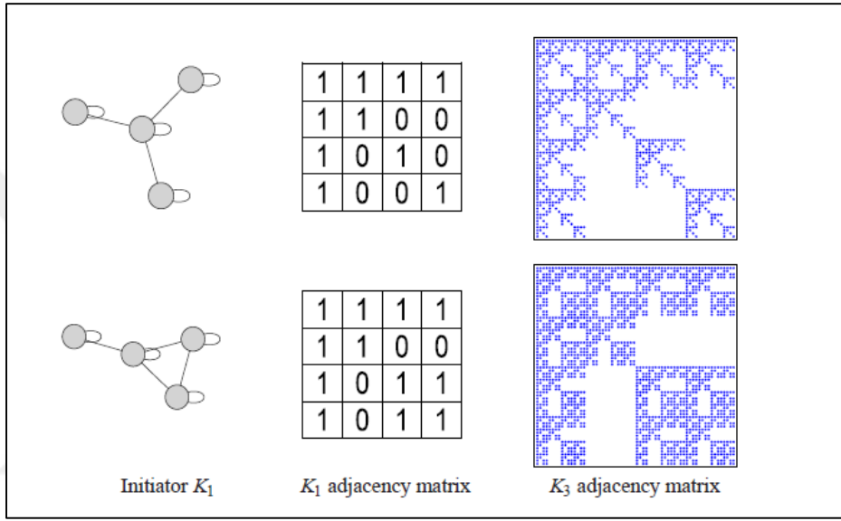
Şekil 2.13. Kronecker çizgelerinde iki farklı başlangıç çizgesi ile başlanarak ağın büyütülmesi sonucu oluşan ağa ait komşuluk matrisi [40].
