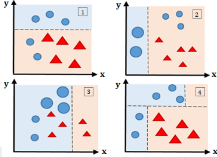
Şekil 2.7. Adaboost Algoritması [62]
