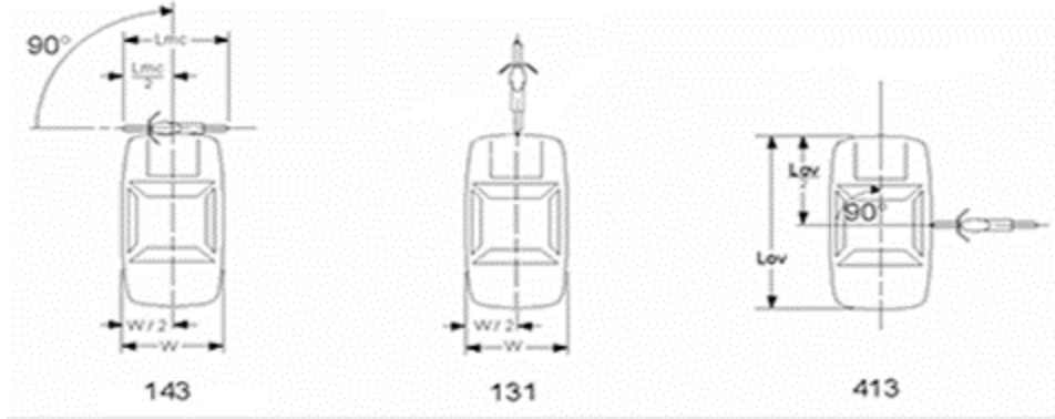
Şekil 2.15. ISO13232'ye göre dört tekerlekli scooter için çarpışma senaryoları [3]
