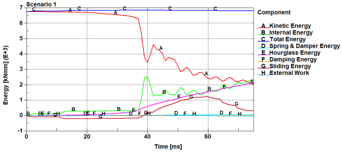
řekil 5.1. Durum 1 için enerji dengesi
