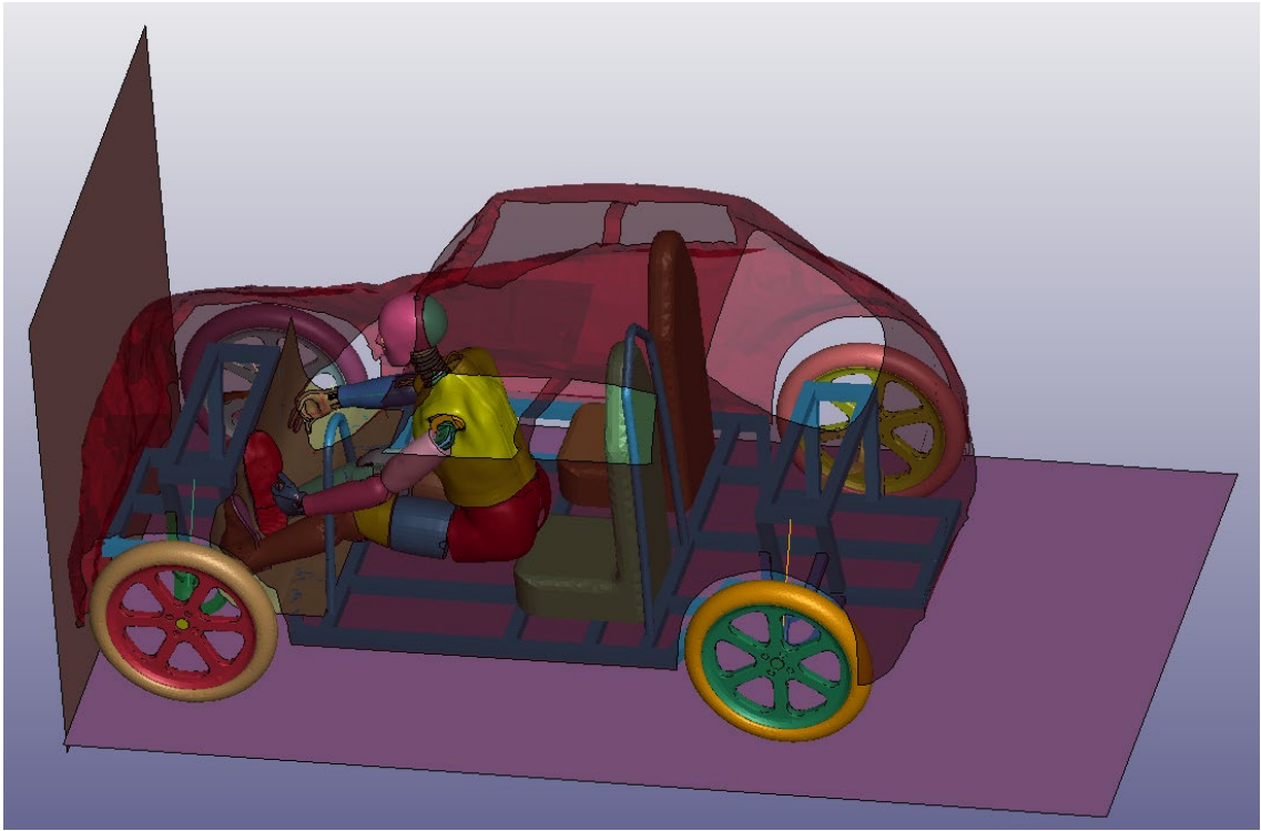
Şekil 4.13. Analiz sonu model görüntüsü (durum 3)
