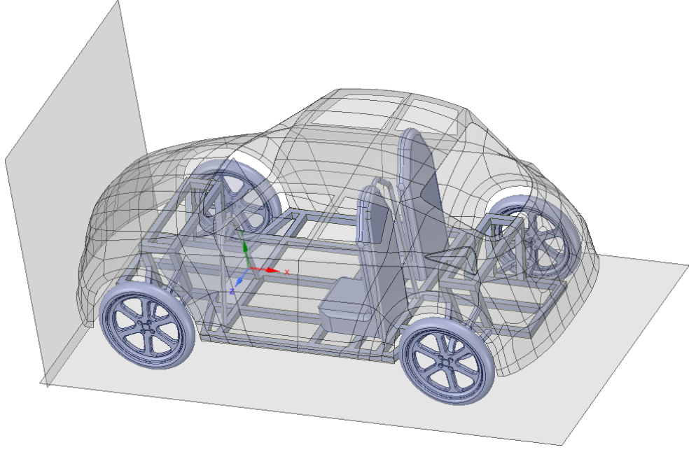
Şekil 3.3. Düzenlenen model görüntüsü
