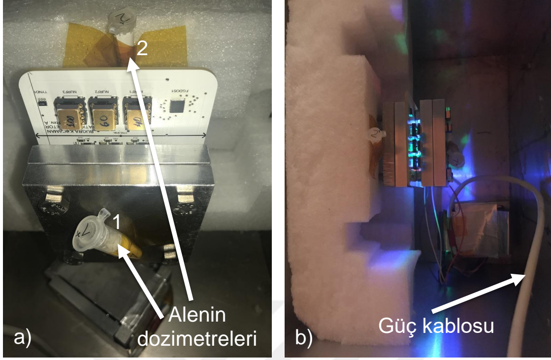
Şekil 3.19. a) Alenine dozimetreleri, b) dedektörün güç kabloları ile enerji verilerek çalıştırılmış hali
