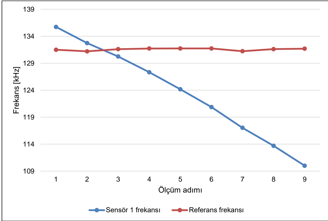
Şekil 4.3. Tedarik edilen tarihçeli FGDOS içerisinde yer alan Sensör 1'e ait ölçüm sonuçları
