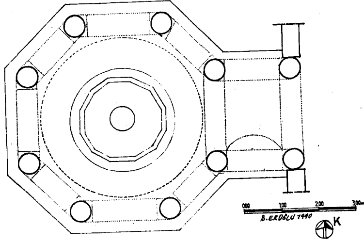
İZMİR ŞADIRVAN ALTI CAMİİ ŞADIRVAN PLANI ÇİZİM. 28
