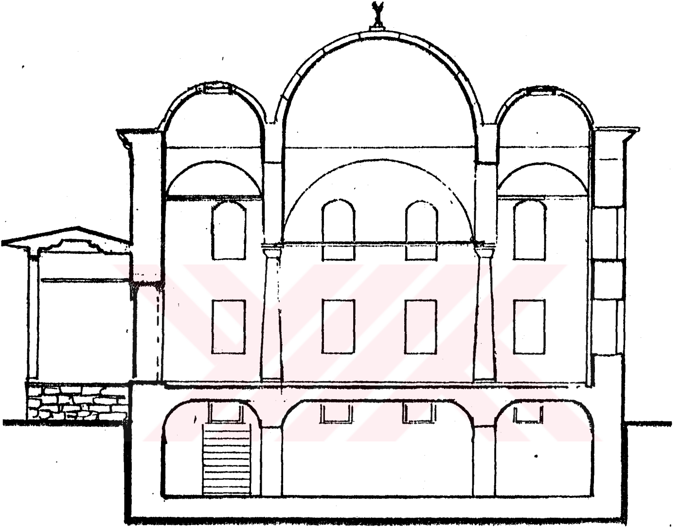
ÇİZİM. 46 MURAT MOLLA KÜTÜPHANESİ KESİTİ (R.S. ATILGAN'dan tadilen)
