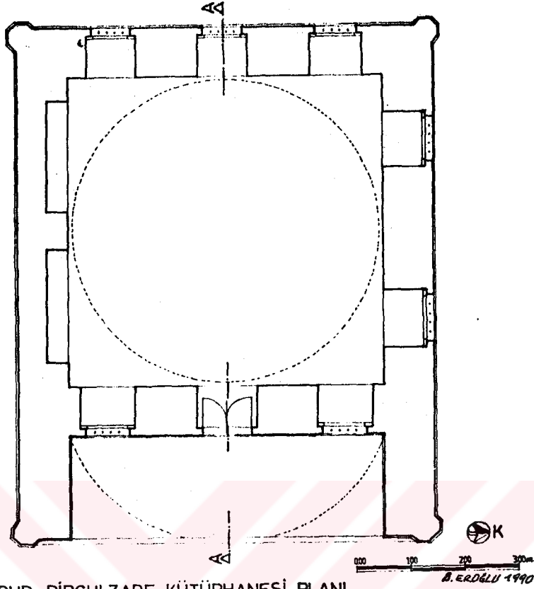
BURDUR PİRGULZADE KÜTÜPHANESİ PLANI
