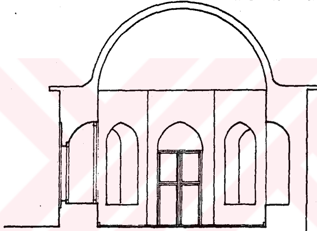
ÇİZİM. 59 AFYON YENİ CAMİİ MUVAKKİTHANESİ KESİTİ
