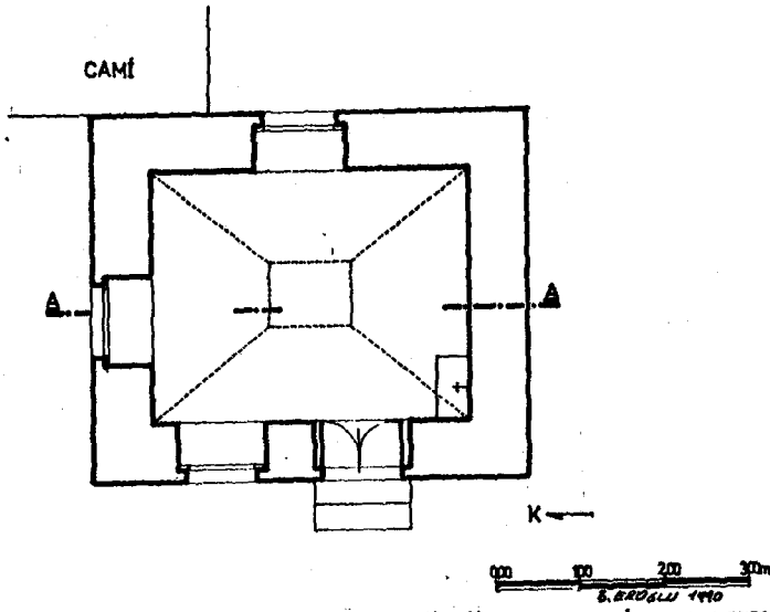
ÇİZİM. 32 AFYON YENİ CAMİ KÜTÜPHANESİ PLANI
