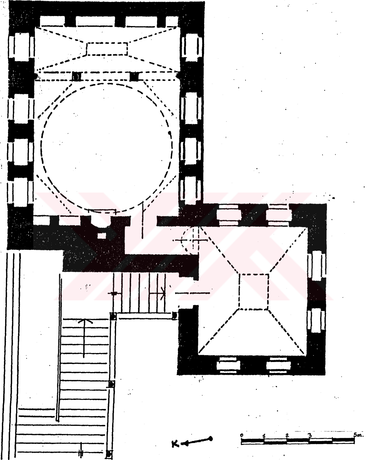
ÇİZİM. 53 ŞEHİT ALİ PAŞA KÜTÜPHANESİ PLARI (B.ÜNSAL'den)
