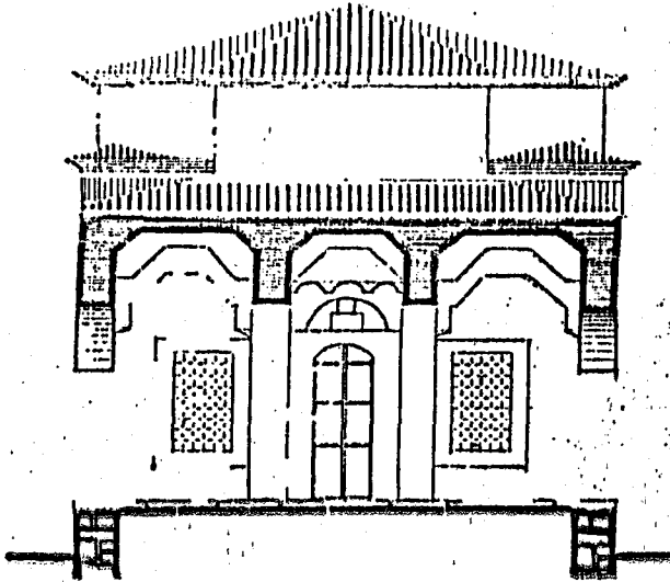
İZİM. 12 AKHISAR ZEYNELZADE KÜTÜPHANESİ KESİTİ(S.KARAGÖZ'den)
