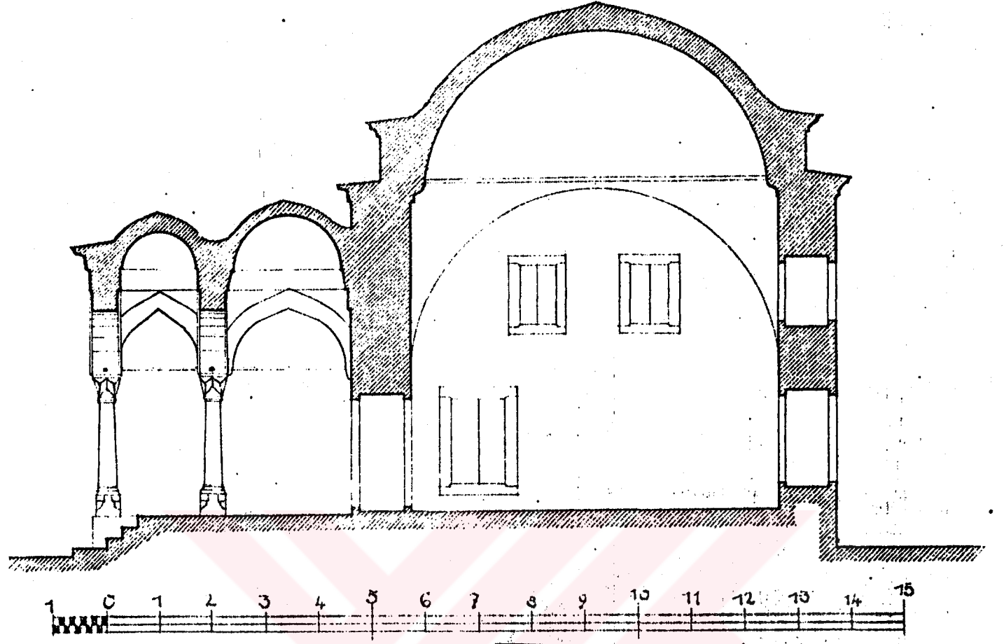
ÇİZİM. 38 KÖPRÜLÜ KÜTÜPHANESİ KESİTİ (Y.ÖNGE'den)
