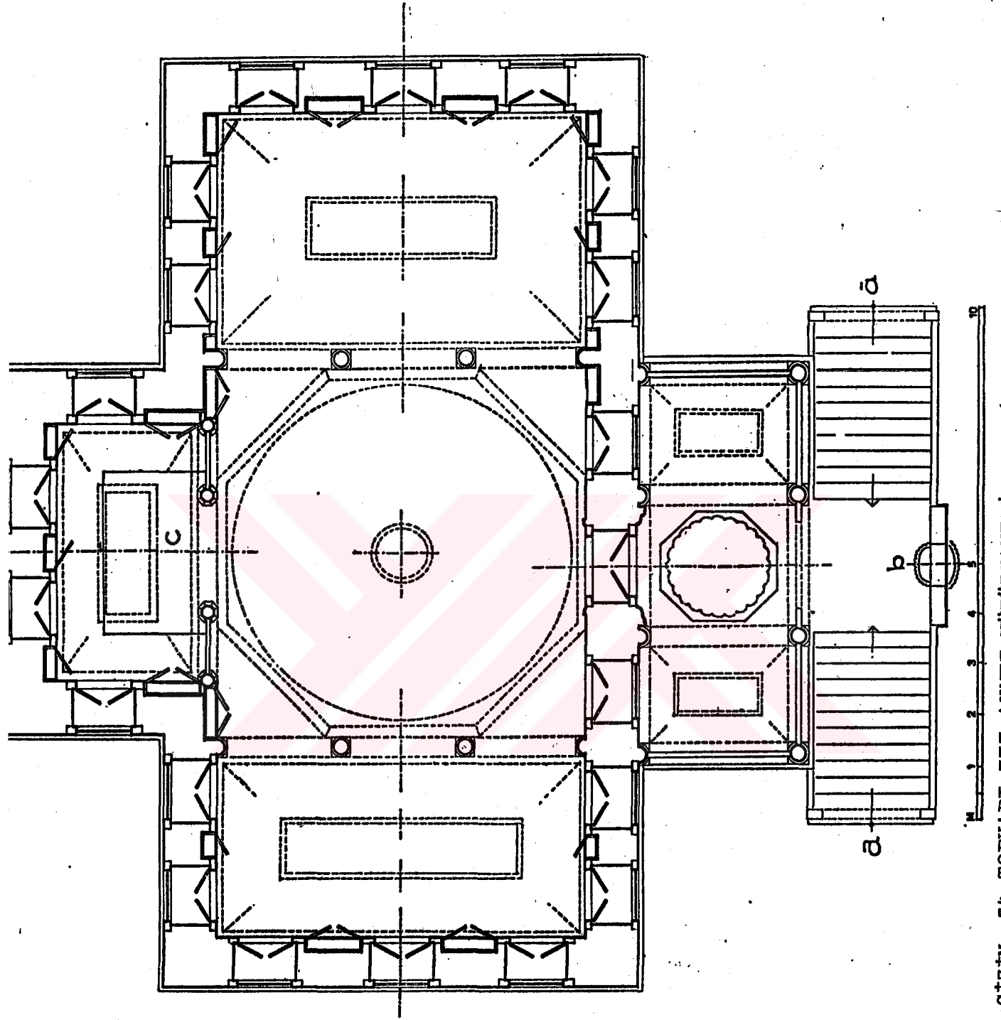
ÇİZİM. 54 TOPKAPI III.AHMET KÜTÜPHANESİ PLANI (S.H. ELDEM'DEN)
