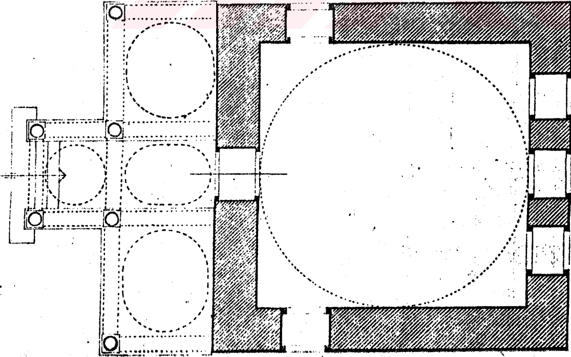
ÇİZİM. 39 KÖPRÜLÜ KÜTÜPHANESİ PLANI (Y.ÖNGE'den)
