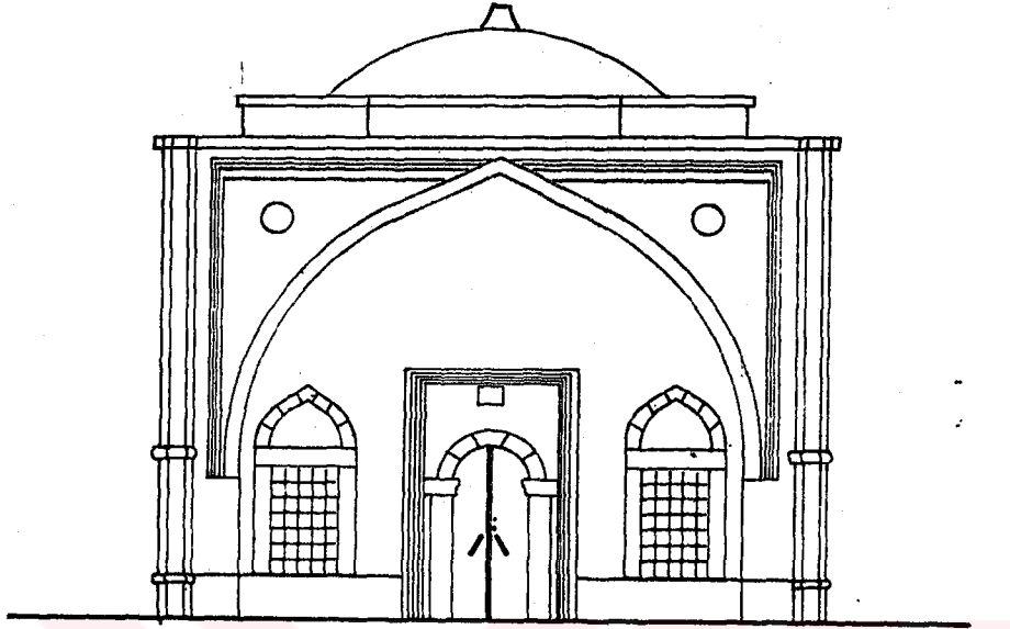
BURDUR PİRGULZADE KÜTÜPHANESİ DOĞU CEPHESİ
