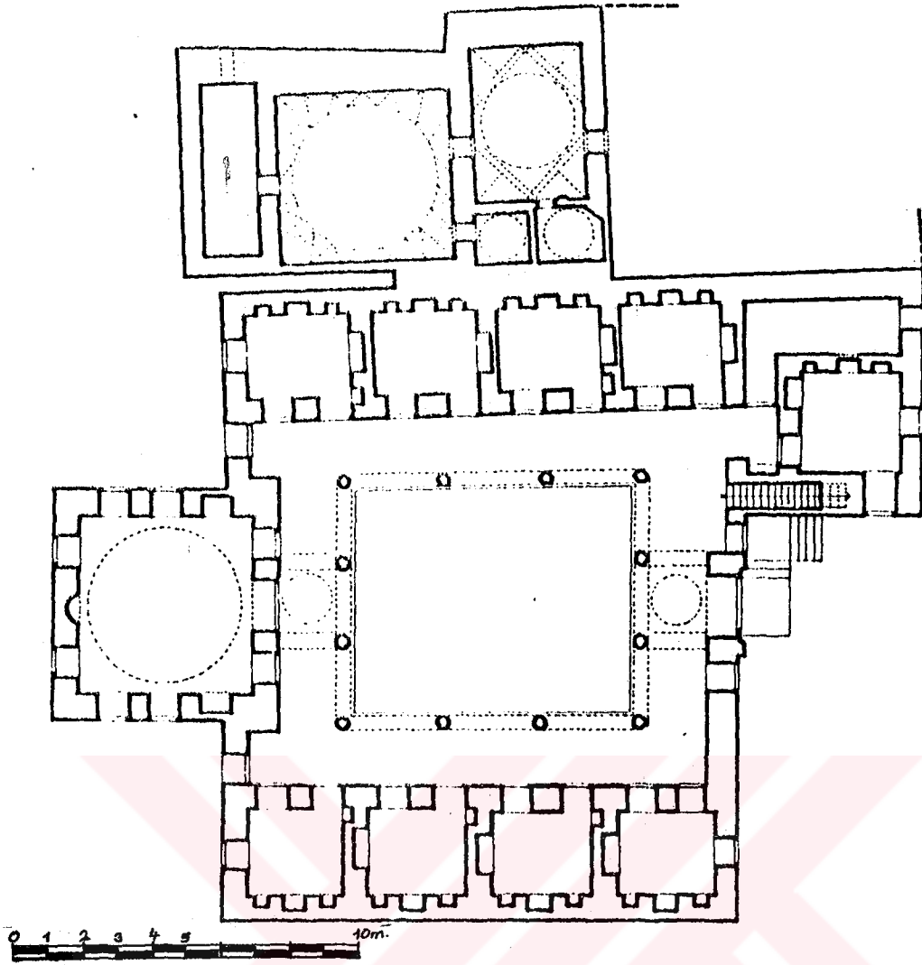
ÇİZİM. 43 SUBAŞI MEDRESESİ PLANI
