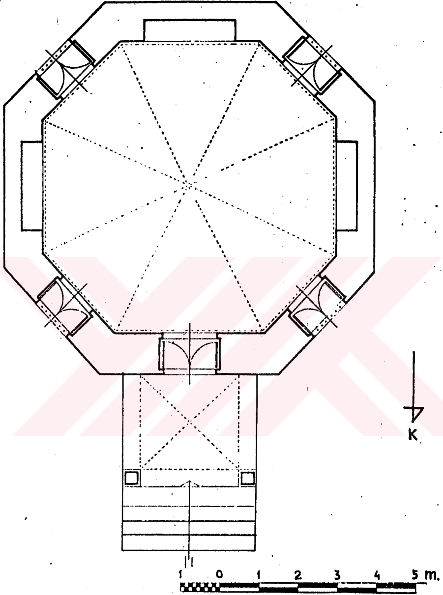
ÇİZİM. 14 MANİSA MURADIYE KÜTÜPHANESİ PLANI (S. KARAGÖZ'den)
