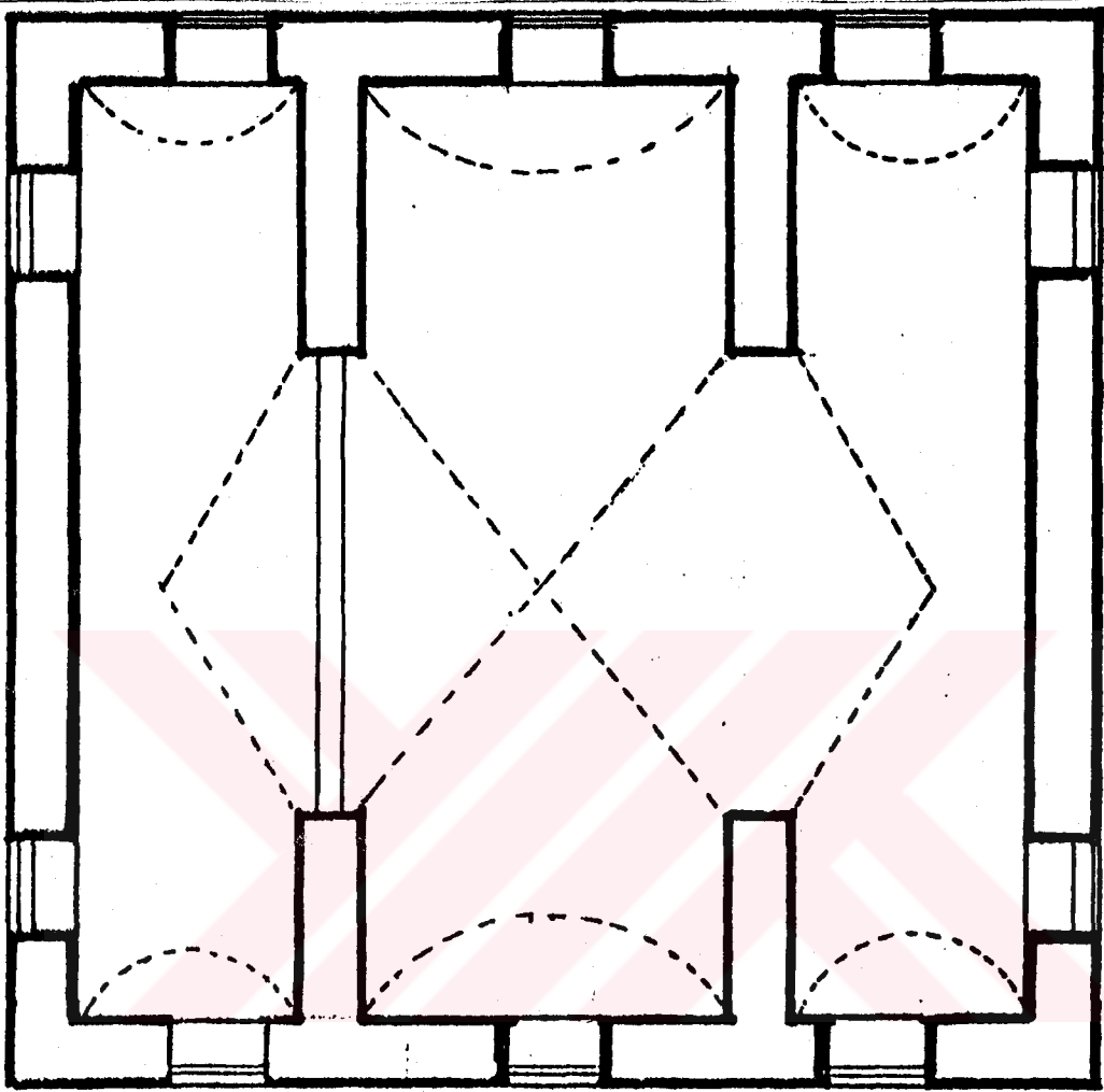
ÇİZİM. 44 MURAT MOLLA KÜTÜPHANESİ BODRUM PLANI (R.S. ATILĞAN'dan)
