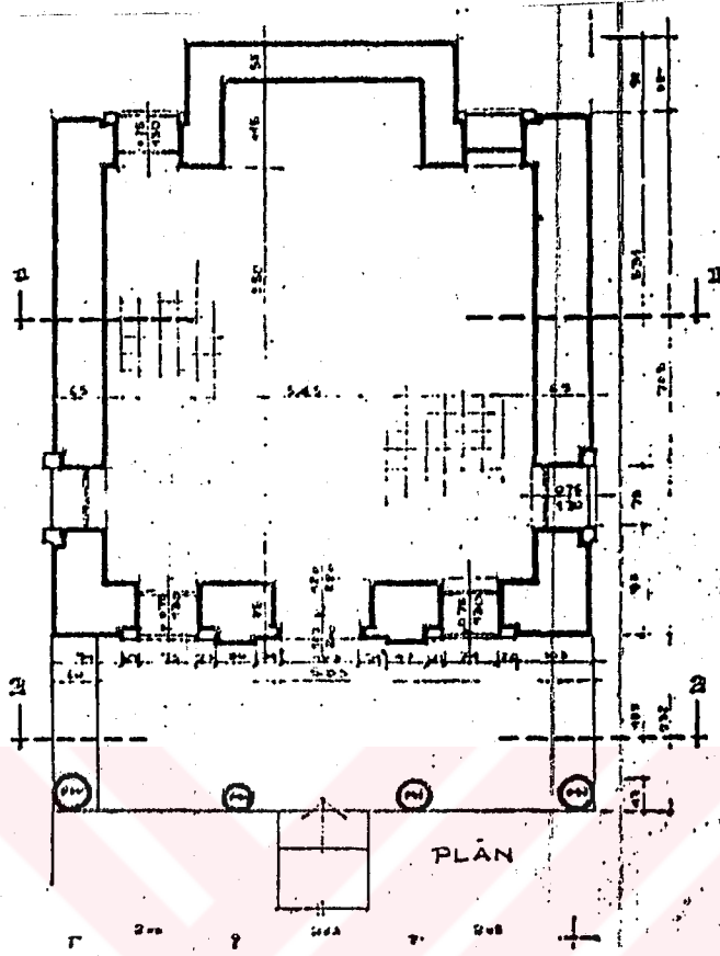
ÇİZİM. 11 AKHISAR ZEYNELZADE KÜTÜPHANESİ PLANI(S.KARAGÖZ'den)
