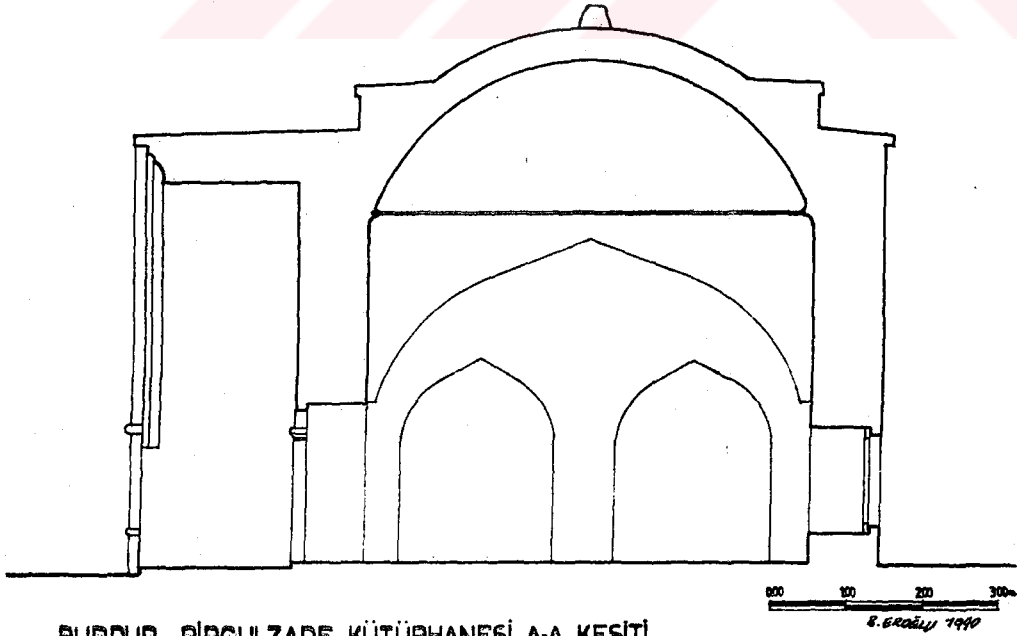
BURDUR PİRGULZADE KÜTÜPHANESİ A-A KESİTİ
