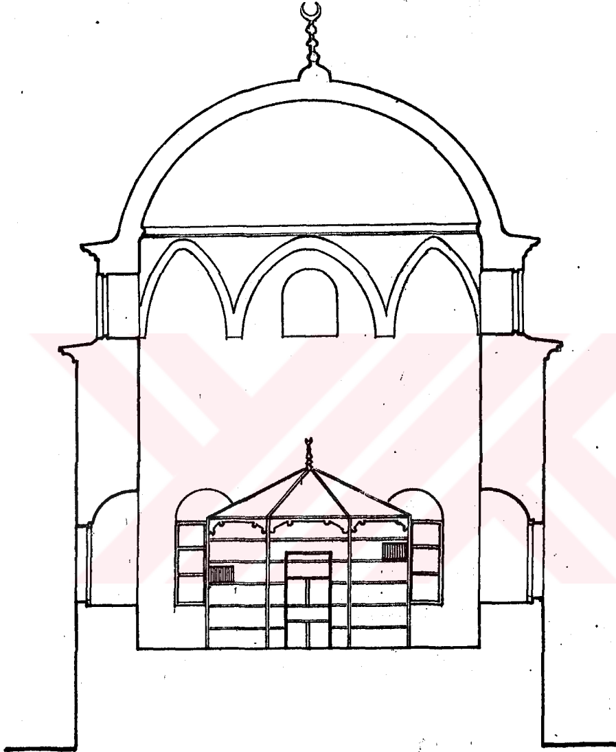
NECİP PAŞA KÜTÜPHANESİ A-A KESİTİ
