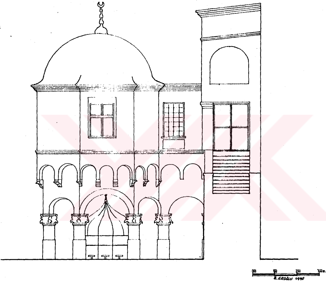
İZMİR ŞADIRVAN ALTI CAMII KÜTÜPHANESİ GÜNEY CEPHESİ
