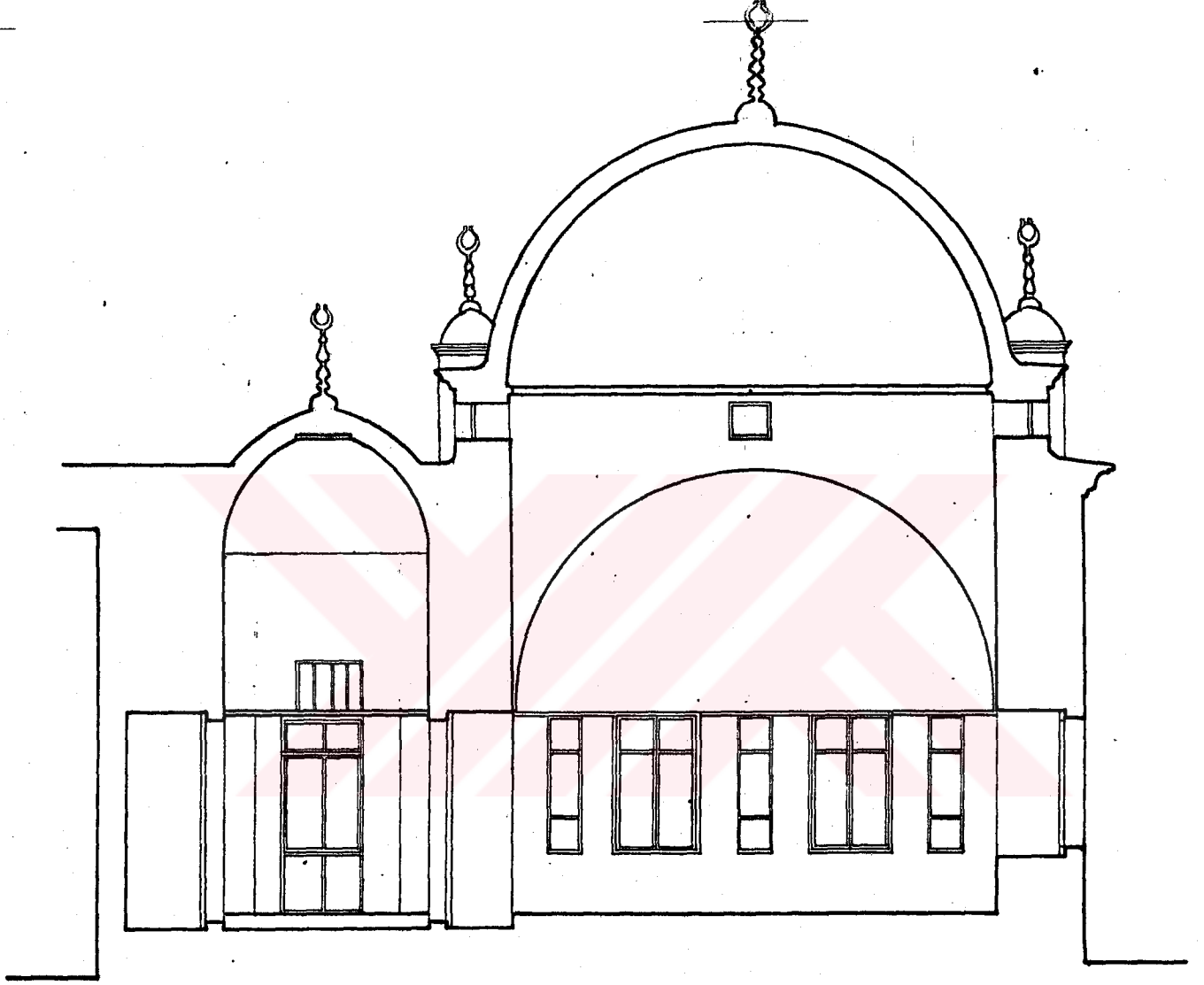
RASİT EFENDİ KÜTÜPHANESİ BOY KESİTİ
