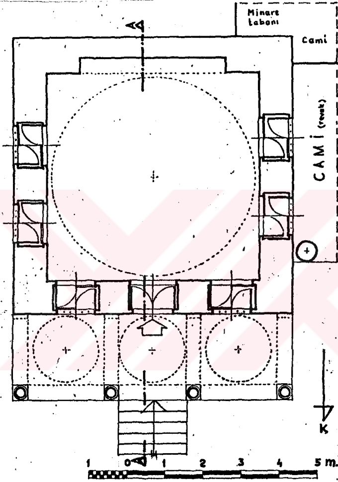
ÇİZİM. 25 MANİSA ÇEŞNİĞİR KÜTÜPHANESİ PLANI(S.KARAGÖZ'den tadilen)
