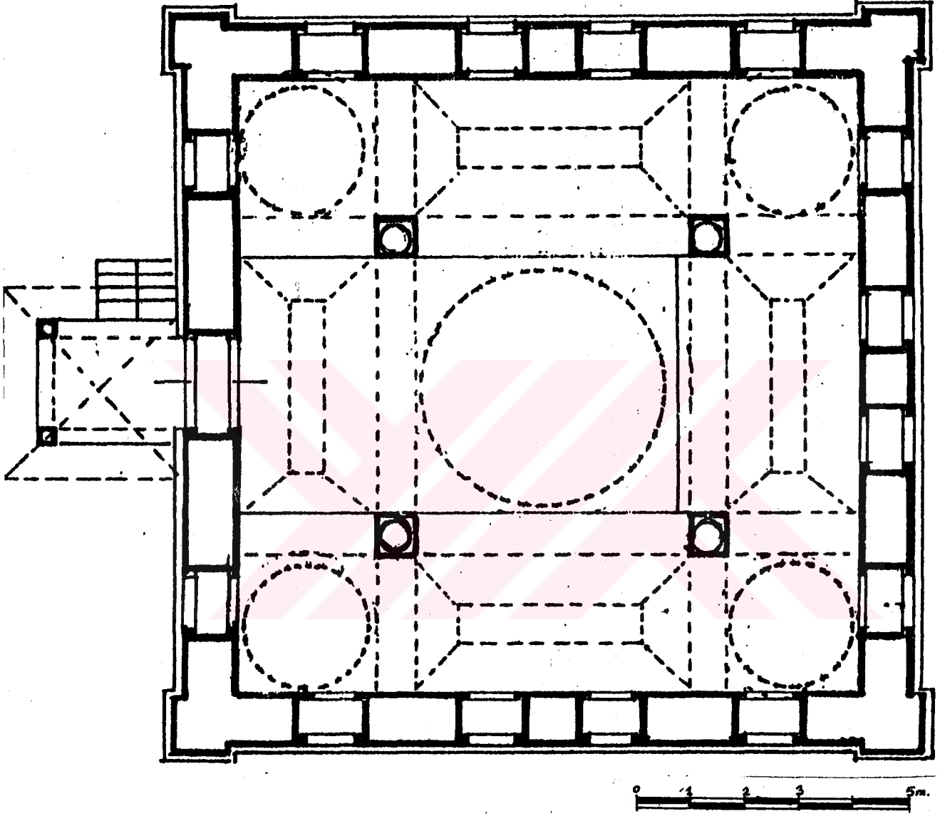
ÇİZİM. 45 MURAT MOLLA KÜTÜPHANESİ PLANI (R.S. ATILĞAN'dan)
