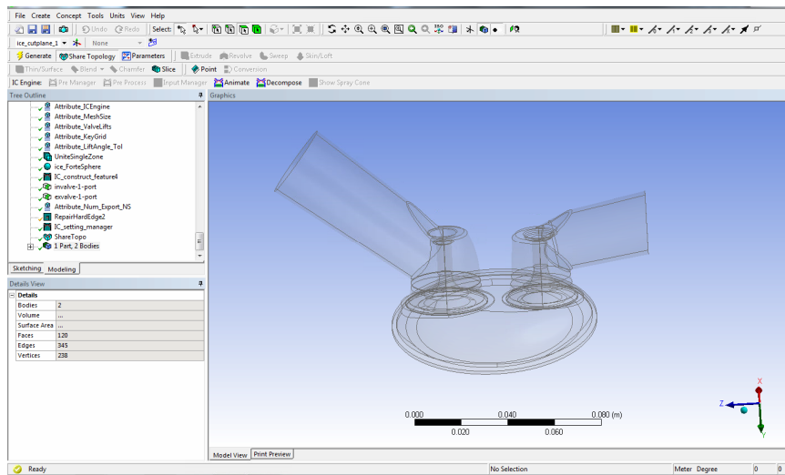
Şekil 5.8. Parçalara ayırma işlemi gerçekleştikten sonraki geometrinin görünümü
