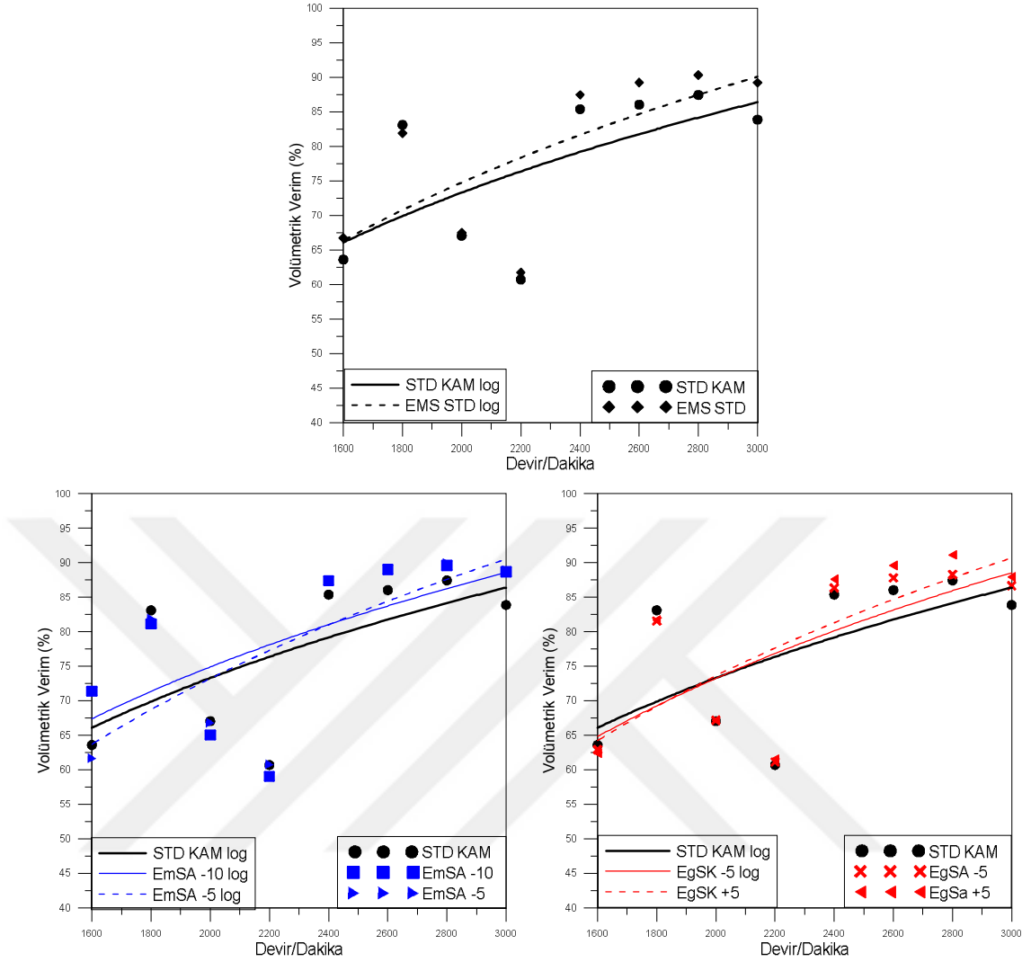
Şekil 7.13. Volümetrik verimin motor hızına göre değişimi
