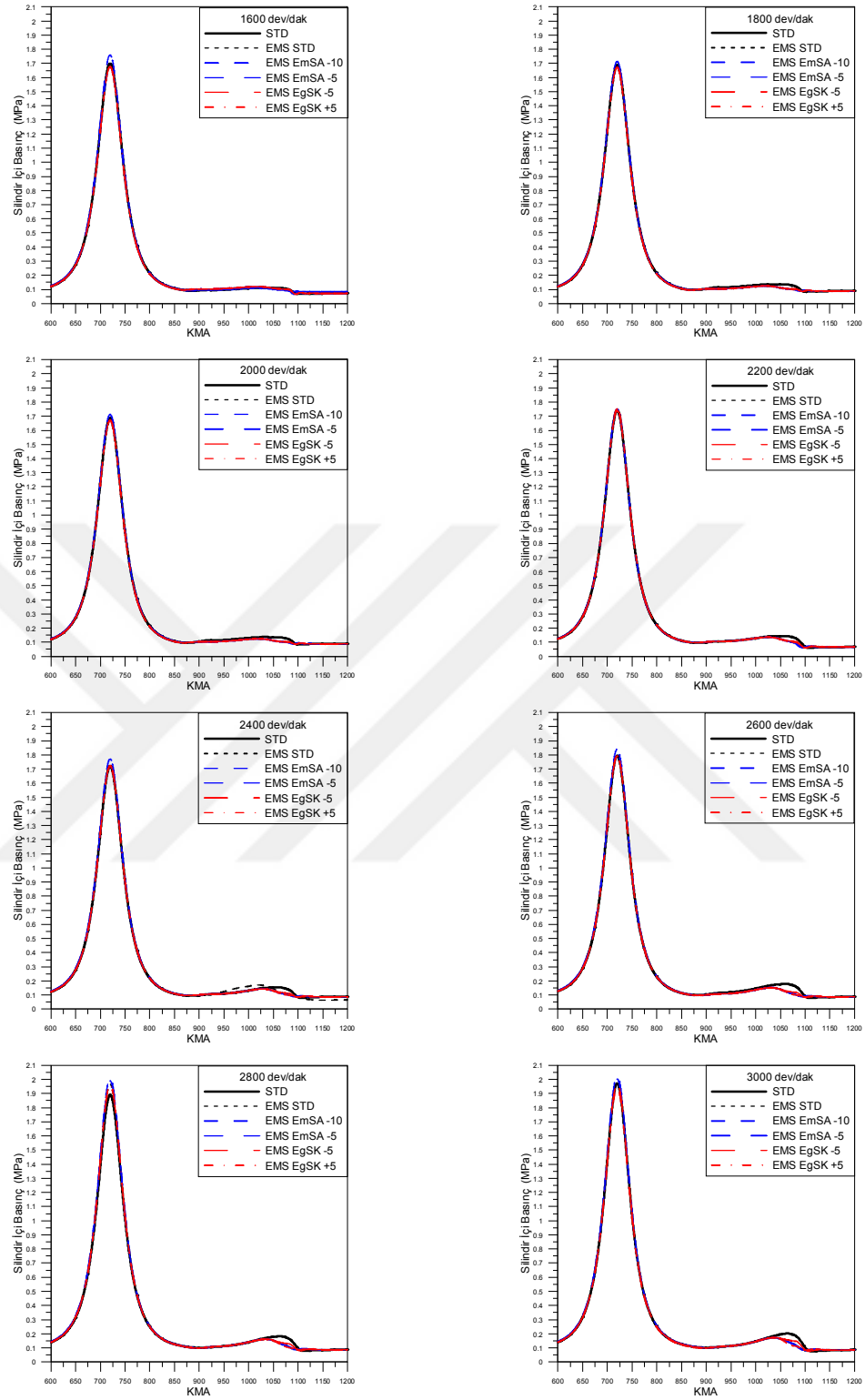
Şekil 7.8. Silindir İçi Basınç Grafiği
