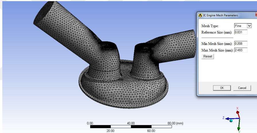
Şekil 5.9. Ağ yapısı parametrelerinin ayarlanması
