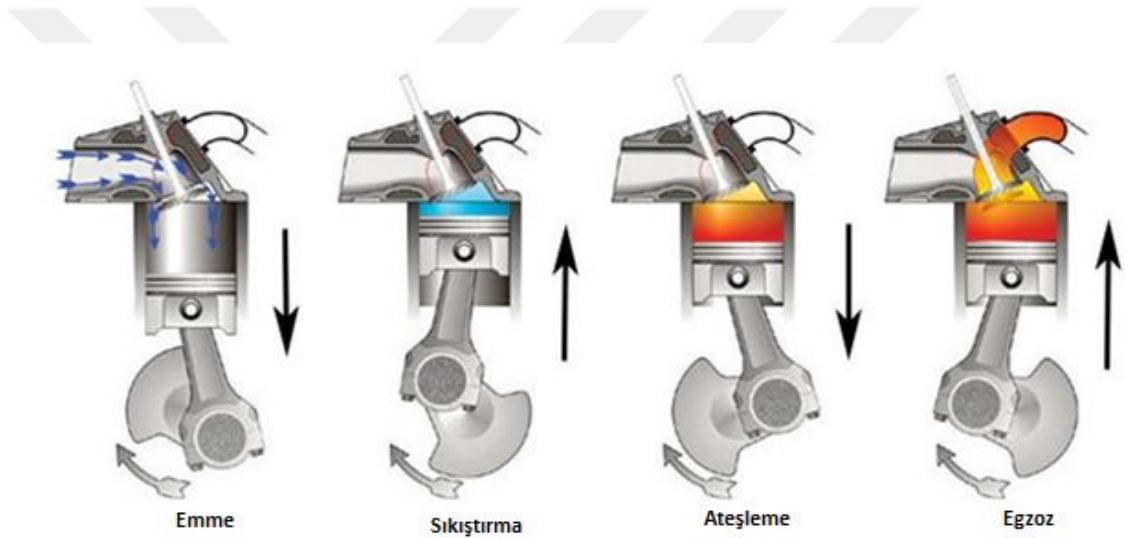
Şekil 3.1. Dört zamanlı motorun zaman kavramları [66]
