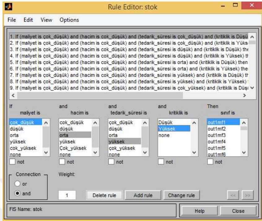
Şekil 4.6. Bulanık Kurallar
