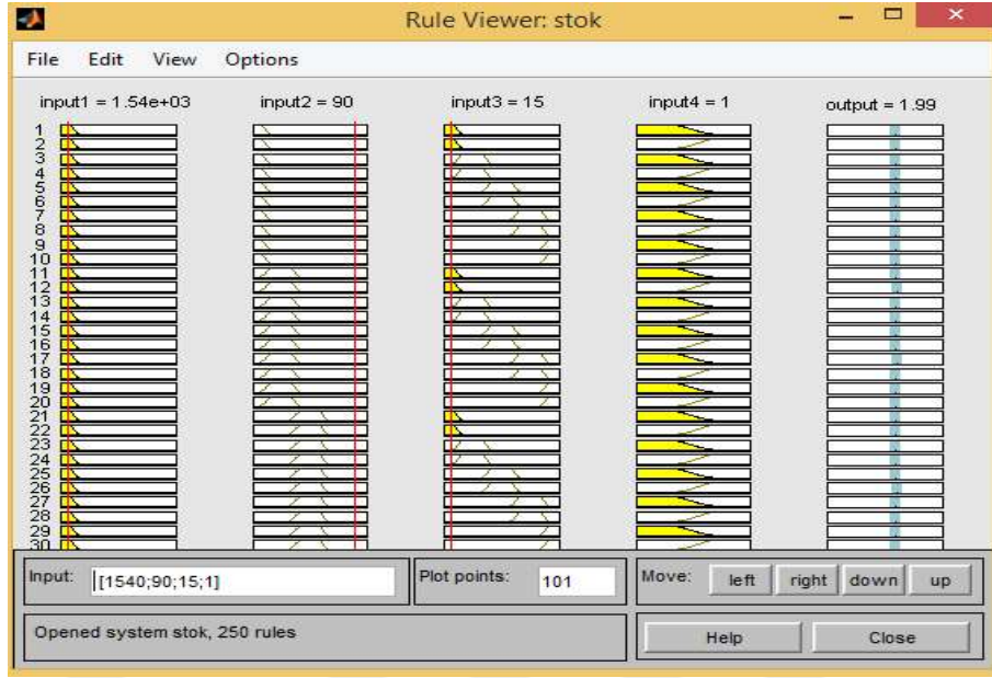
Şekil 4.7. Kural izleyici
