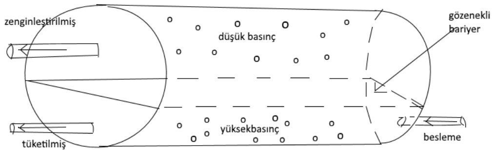
Şekil 3.3. U 235 Bolluk oranı işaretlenmiş gazlı difüzyon aşaması [35].
