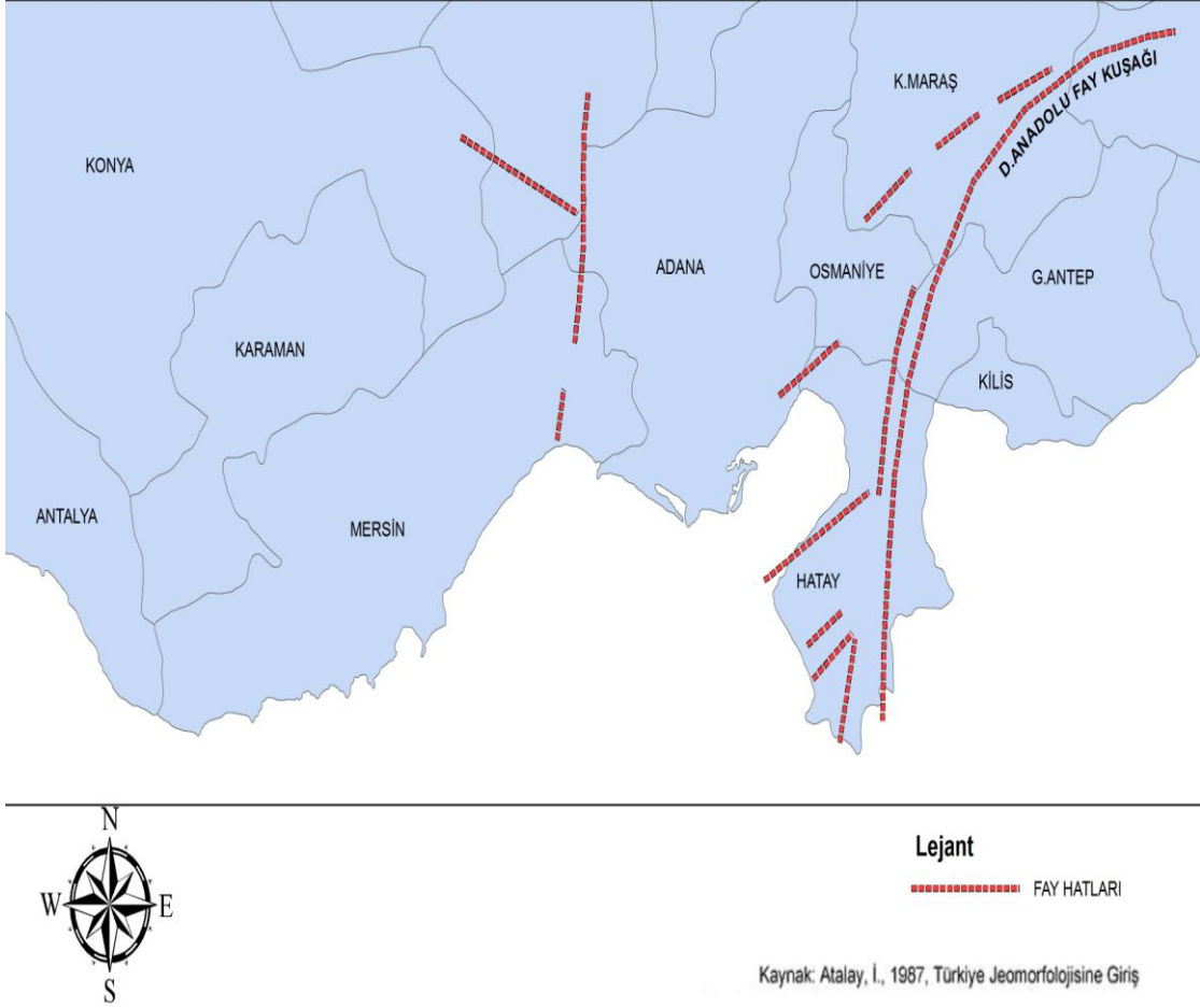
Ek- 13: Çukurova çevresindeki önemli fay hatları.
