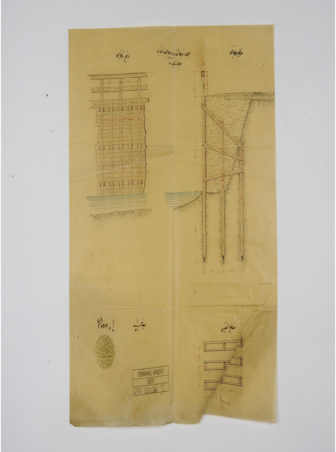
Ek-7: BOA, 1893'te Seyhan Nehri'nin kenarına taşkınları engellemek için yapılacak ahşap settin planı.
