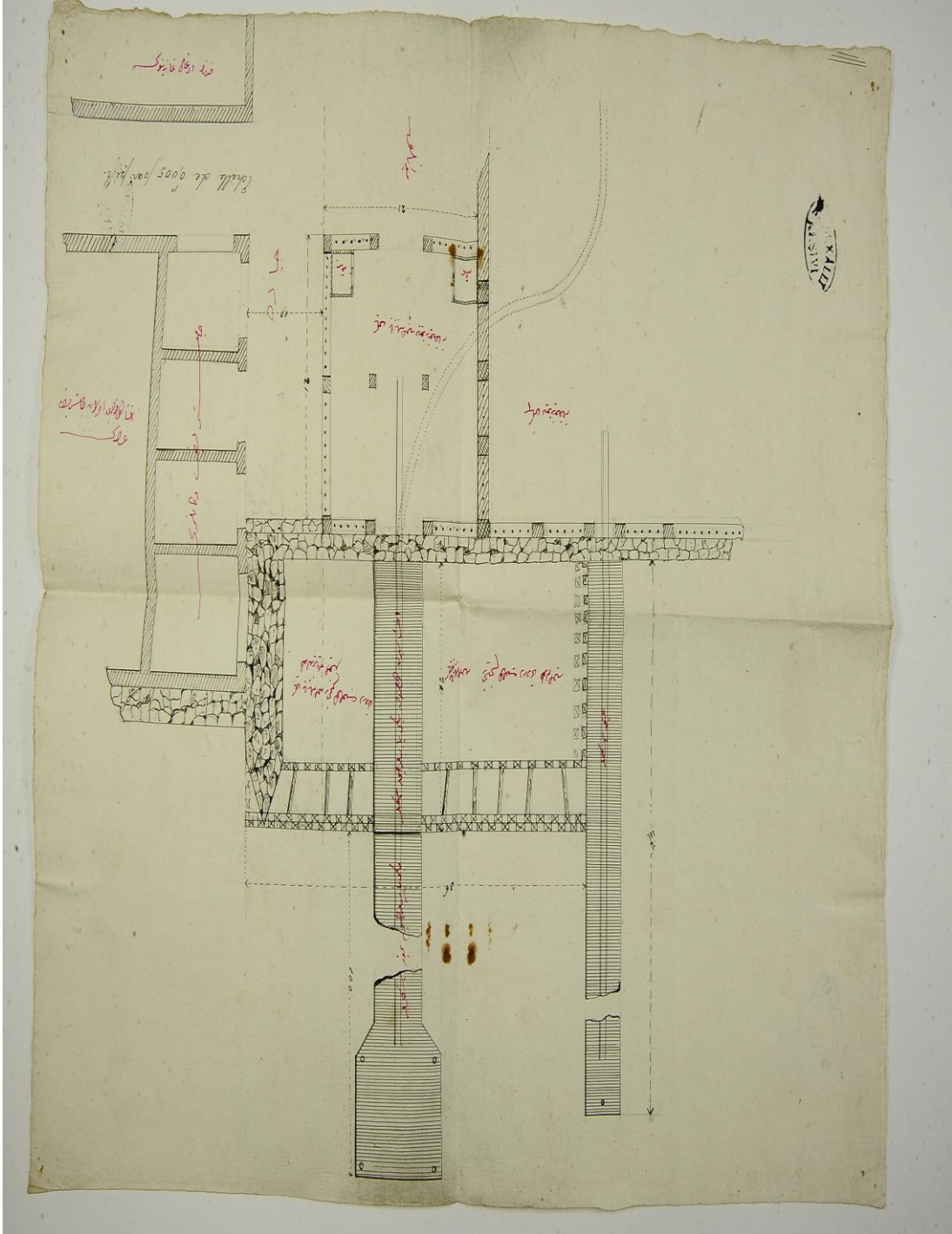
Ek-9: BOA, Mersin'de fırtınadan yıkılan ahşap iskele yerine inşa edilecek demir iskelenin planı.
