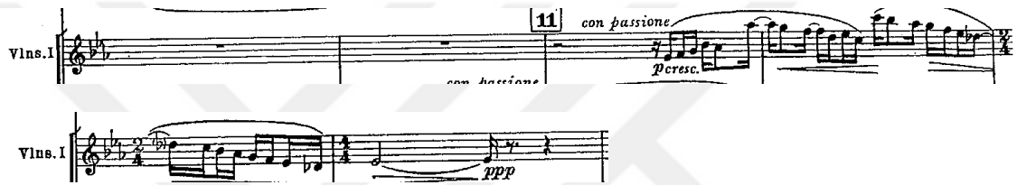
Örnek 31: Bölümün Kapanış Bölmesindeki Ezgisel Hattın Sol Ekseninden Do Eksenine Kaydırılması
