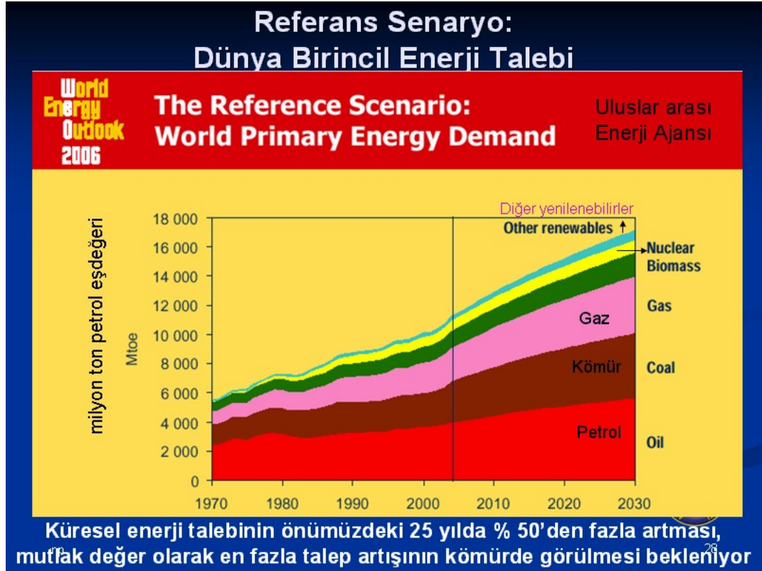
Şekil 5. 1970-2030 Yılları Arasındaki Gerçekleşen ve Tahmini Dünya Enerji Talebi
