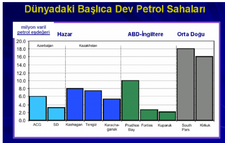
Şekil 6. Dünyanın Büyük Petrol Rezervleri ile Hazar Petrol Rezervlerinin Karşılaştırılması
