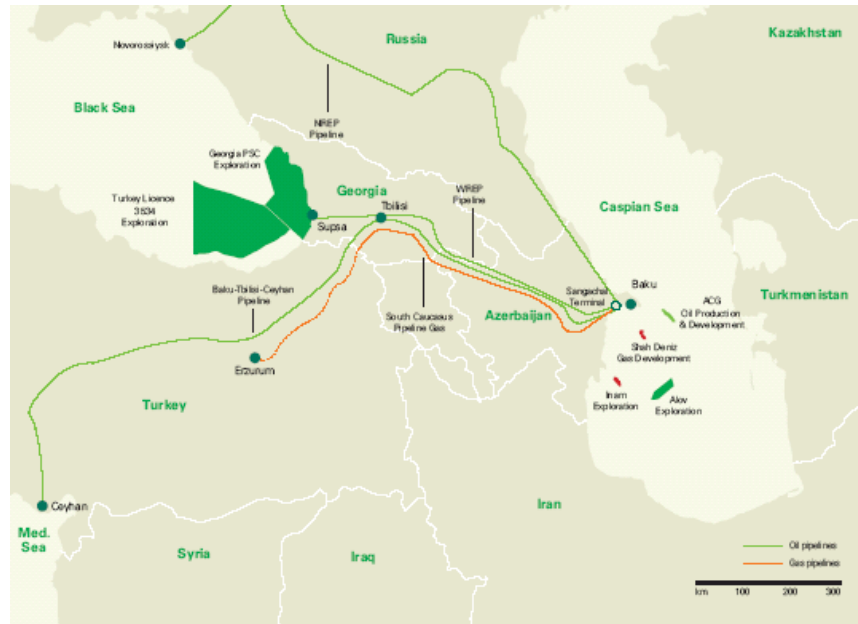
Şekil 3. Azerbaycan'dan Diğer Ükelere Giden Petrol ve Doğal Gaz Boru Hatları
