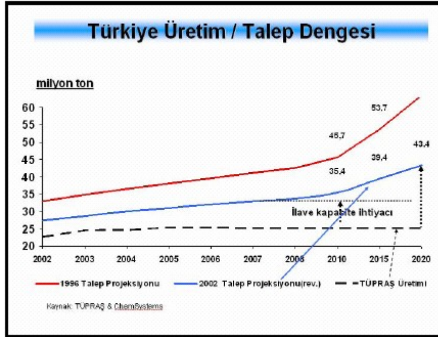
Şekil 8. Türkiye'nin 2002-2020 Yılları Arasındaki Petrol Ürünleri Üretim-Talep Dengesi
