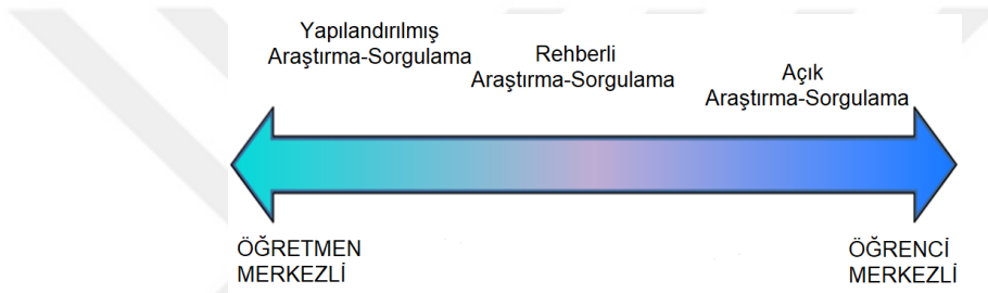
Şekil 1. Araştırma-sorgulama düzeyleri.
