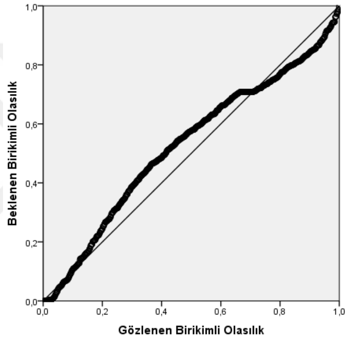
Şekil 2. Beklenen ve gözlenen birikimli olasılık.
