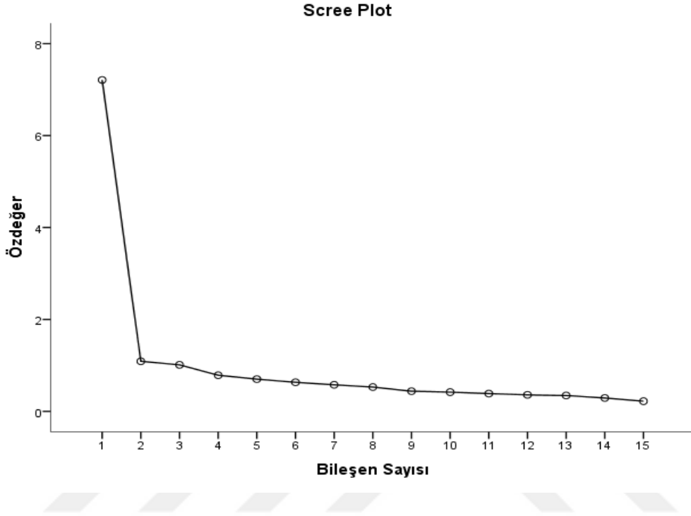
Şekil 4. ÖÖÖ serpilme diyagramı (scree plot).
