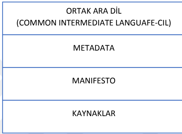
Şekil 14: .NET Assembly
