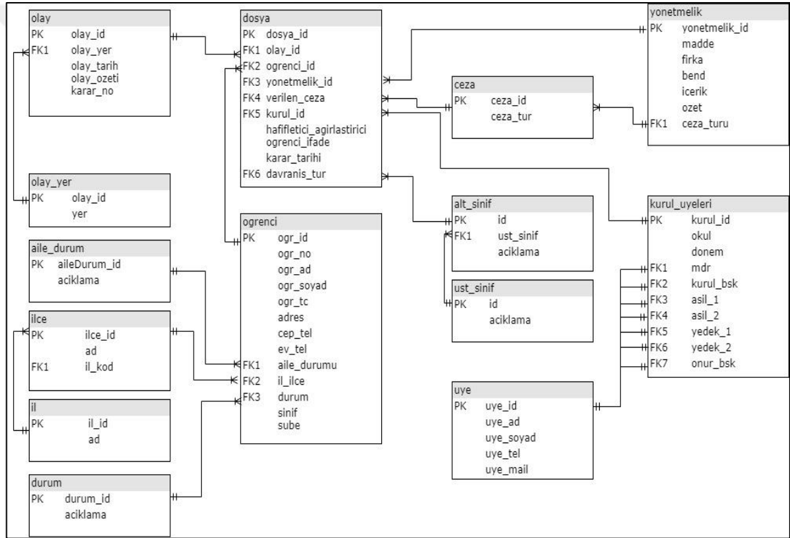
Şekil 8: İlişki Diyagramı
