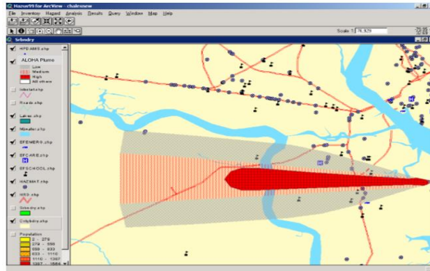
Resim 1: ALOHA Hava Kaplaması HAZUS Envanteri
