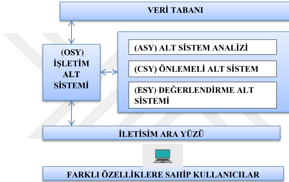
Şekil 10: RODOS Sisteminin Kavramsal Yapısı
