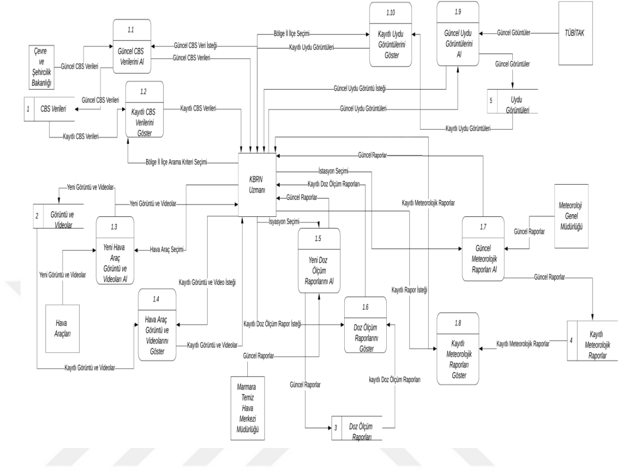
Şekil 17: Veri İzleme Çocuk Diyagramı
