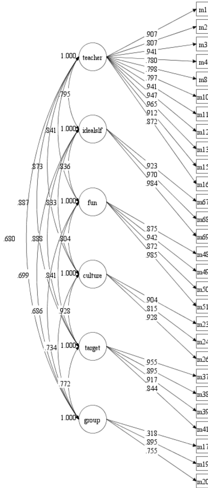
Şekil 2. Ölçme Modeli
