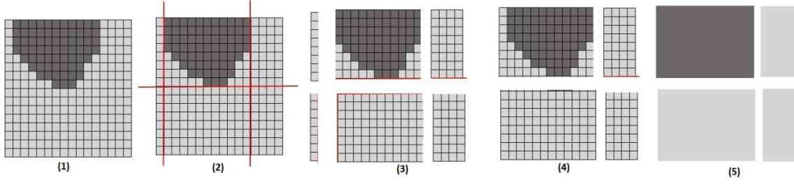
Şekil 3.9. Zon bazlı bölümlenme algoritmasının çalışması
