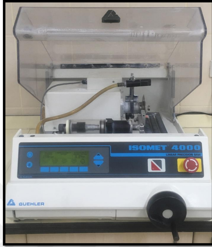
Şekil 3. 7. Çalışmada kesit alma aşamasında kullanılan Isomet 4000 cihazı
