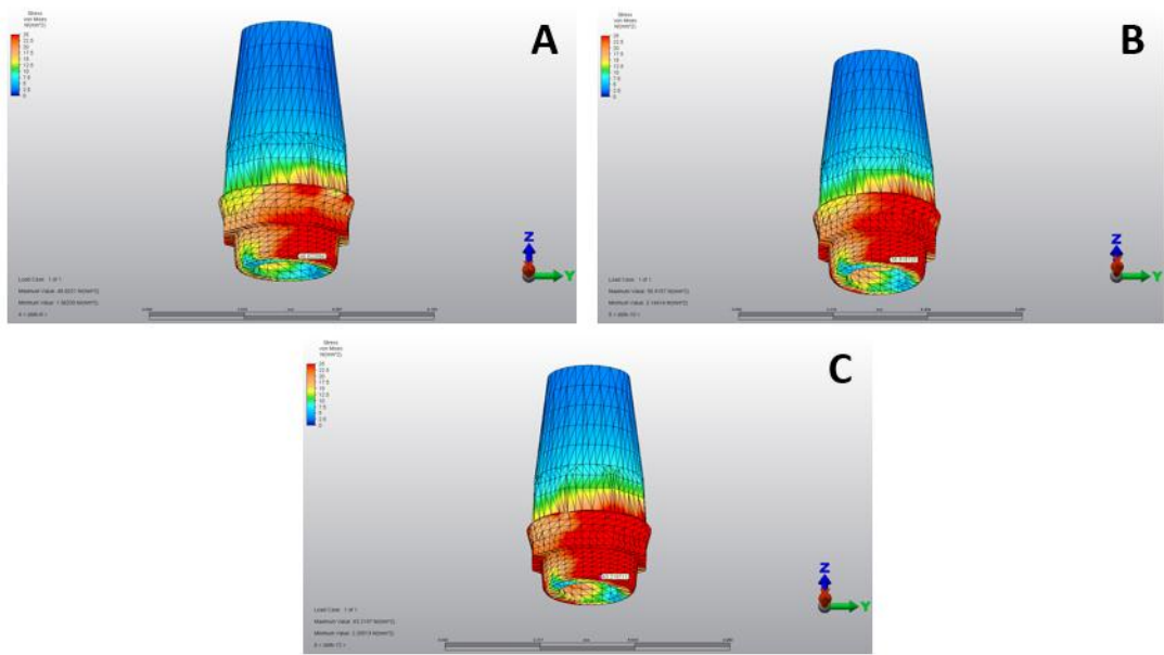
Şekil 4.10. Oblik yükleme ile Model 2’de abutment üzerinde oluşan Von Mises stres dağılımının incelenmesi. A) 8 mm kron yüksekliği mesafesi; B) 10 mm kron yüksekliği mesafesi; C) 12 mm kron yüksekliği mesafesi
