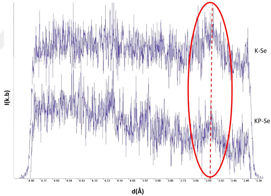
Şekil 4.5. KP ve K gruplarına ait WAXS profilleri
