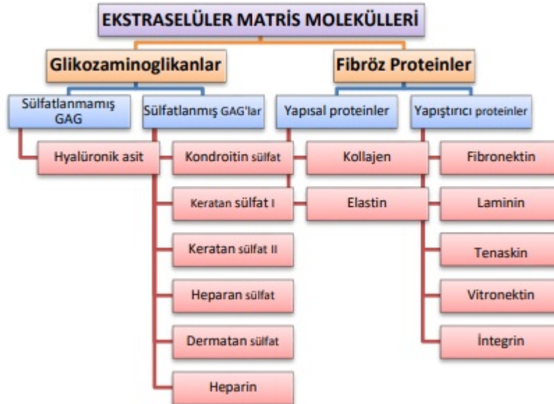
Şekil 2.5. ECM molekülleri
