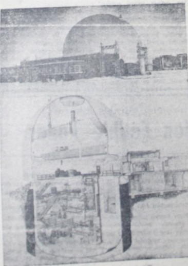
Birleşik Amerikada Argonne Millî Laboratuvarında inşa edilen ve sonunda çalışan bir enerji merkezi, 20.000 kilovatt besleme ve 5.000 kilovatt elektrik tahsis etmektedir. Kaynar su vakitleri ile çalışan merkezini binası tamamlanmıştır. İçinde toprak üzerindeki kızgın su ile müferte kaplıdır. (Elsie Foto servisi)
