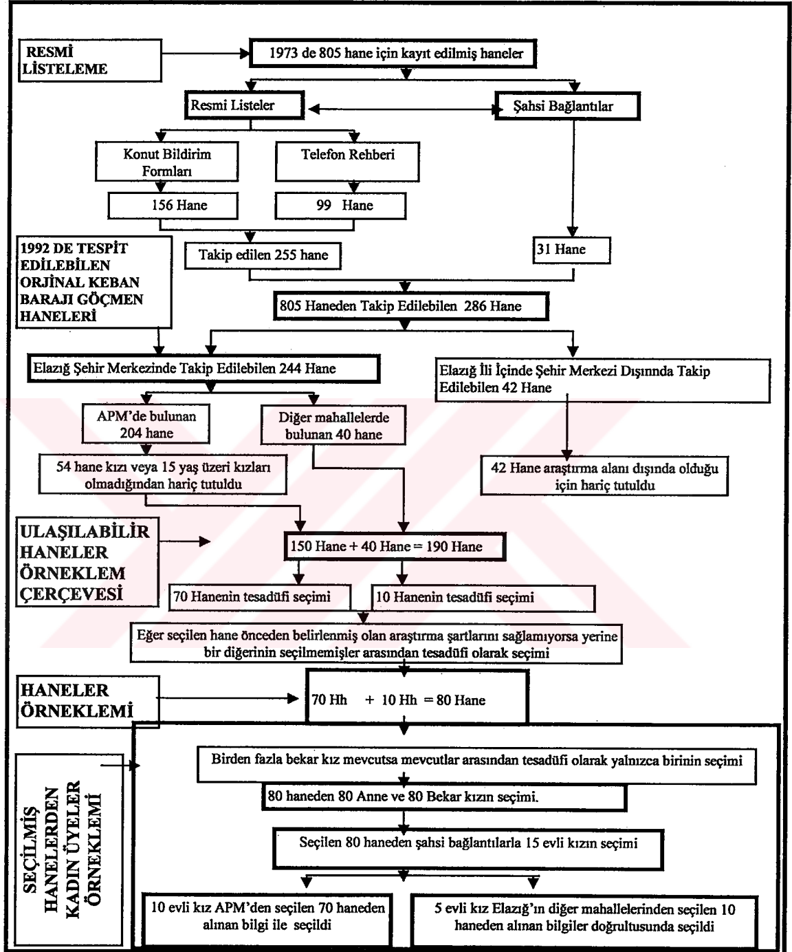
Şekil 3.3:Örneklem Süreci
