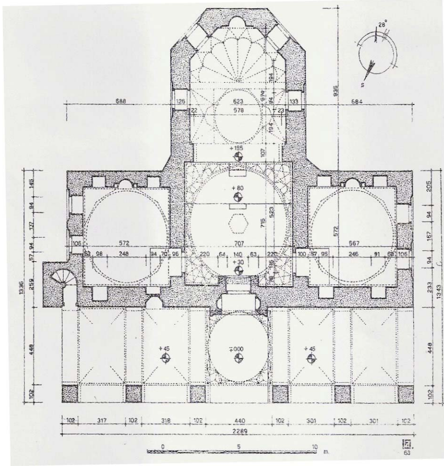
Çizim. 1: Edirne Beylerbeyi Camii Planı ( E.H. AYVERDİ'den)
