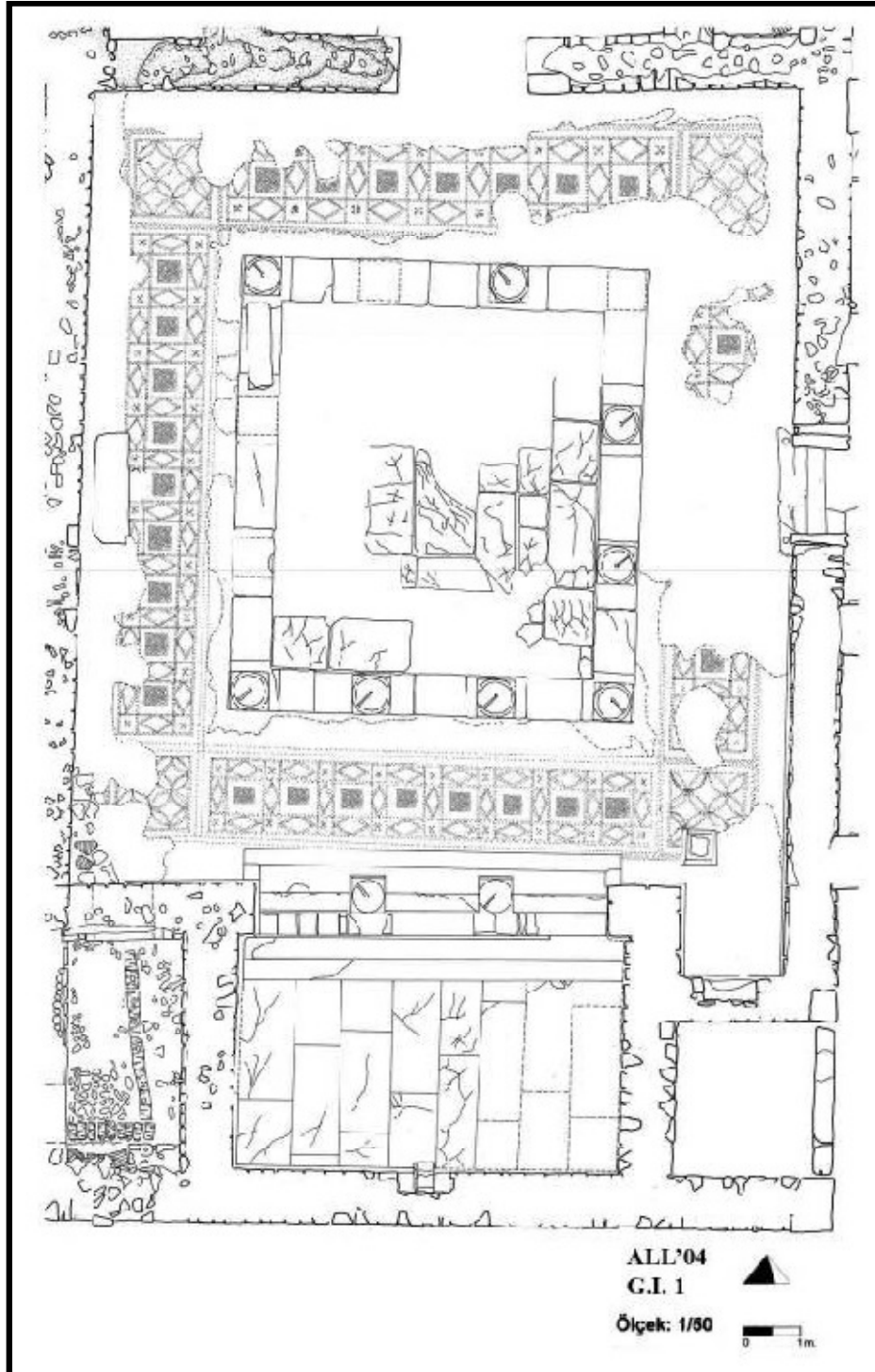
Plan 3 : Frigidarium Plan.
