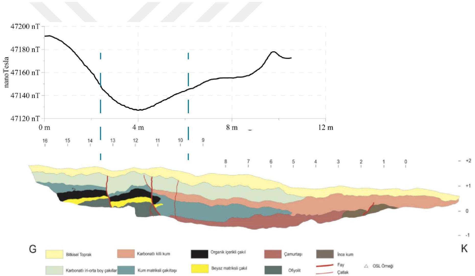
Şekil 4.4. Elde edilen manyetik anomali ve hendek logunun(batı duvarı) karşılaştırması.
