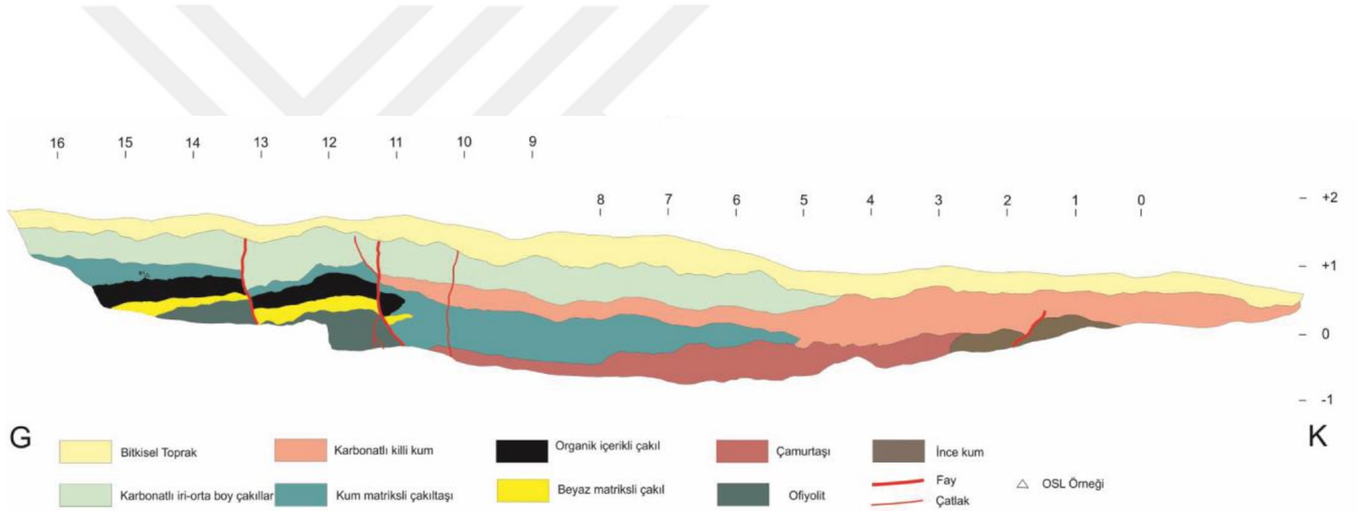
Şekil 3.12. Karabayır hendeği batı duvarı logu.
