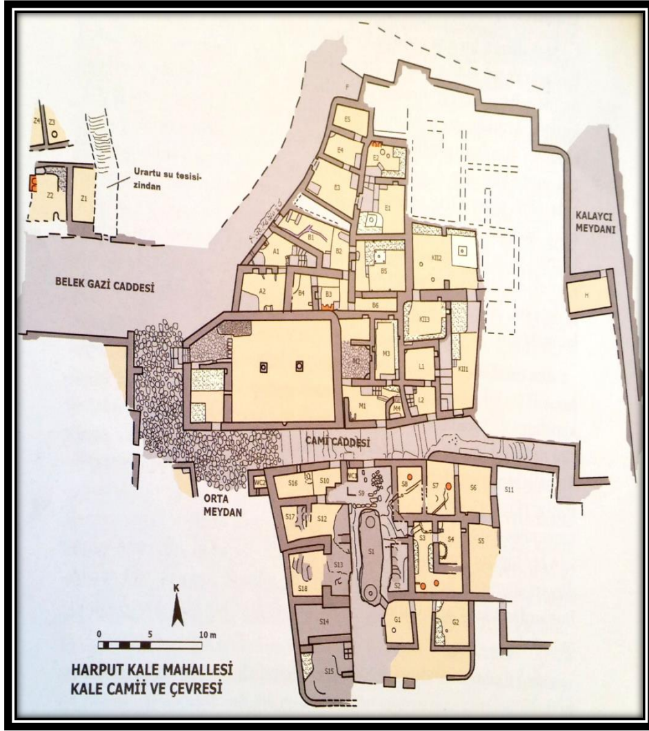
Plan-1: Kale Mahallesinin Merkezi Bölüm Planı (Kaynak: Veli Sevin-Necla Arslan Sevin-Haydar Kalsen, Harput Kale Mahallesinde Osmanlı Yaşamı , s. 106)
