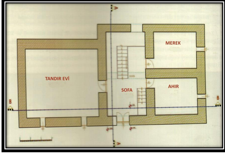
Plan-3: Şefik Gül Evi Zemin Kat Planı (Kaynak: Şahabettin Öztürk, Mithat Coşkun, Geleneksel Harput ve Elazığ Evleri , s. 84.)
