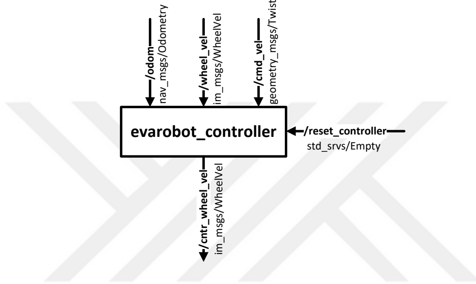
Şekil 3.12 evarobot_controller düğüm yapısı
