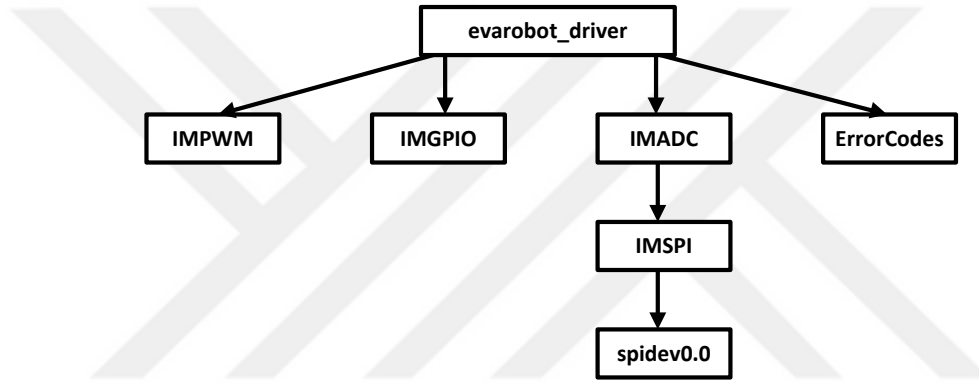
Şekil 3.13 evarobot_driver düğümünün diğer katmanlarla olan ilişkisi
