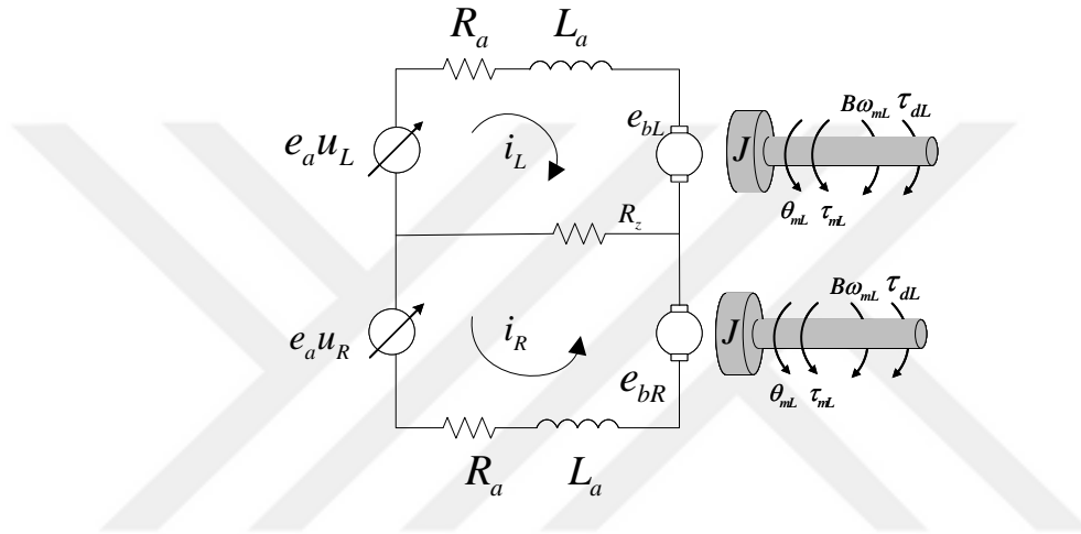
Şekil 3.4 Sağ ve Sol için dc motor modeli
