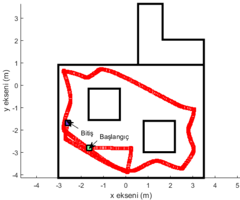
Şekil 4.13 Gerçek ortam rastgele dolaşma davranışı izlenen yörünge
