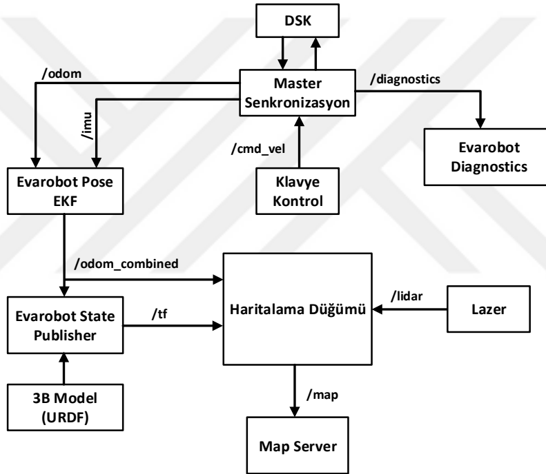
Şekil 3.24 Ortam haritası çıkarılırken kullanılan düğüm yapısı
