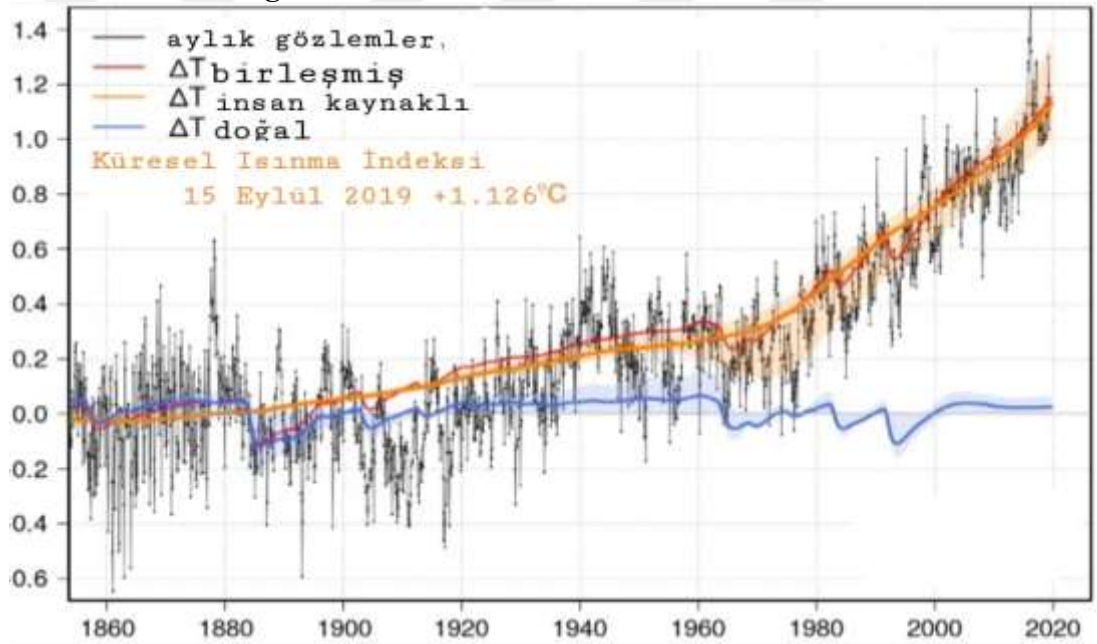
Grafik 18: Yıllara göre küresel ısınma 676
