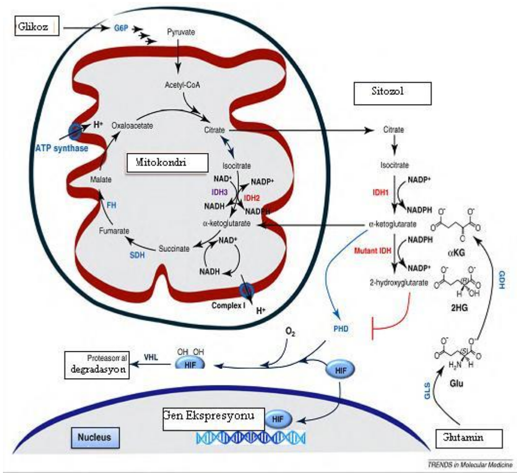
Şekil 2.3. TCA döngüsü ve IDH genleri. TCA siklusundaki enzimler mitokondride ve mutant IDH sitozolde gösterilmiştir. Mutant IDH tarafından 2HG nasıl üretildiği HIF-1α birikimi aracılığı ile PHD (prolyl hidroksilaz) inhibisyonunun kanser gelişimini etkilemesi şematik olarak gösterilmiştir. Kısaltmalar: FH, fumarat hidrataz; SDH, suksinat dehidrogenaz; PHD, prolyl hidroksilaz; GLS, glutaminaz; GDH, glutamat dehidrogenaz; G6P glikoz 6-phosfat (Dang ve arkadaşlarından değiştirilerek alınmıştır.)(18).
