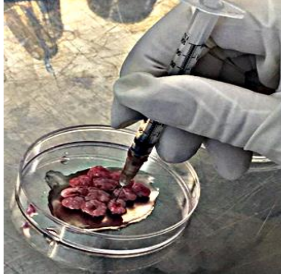
Şekil 5.2. Ovaryumlardaki foliküllerin patlatılarak enzimatik sindirime hazır hale getirilmesi
