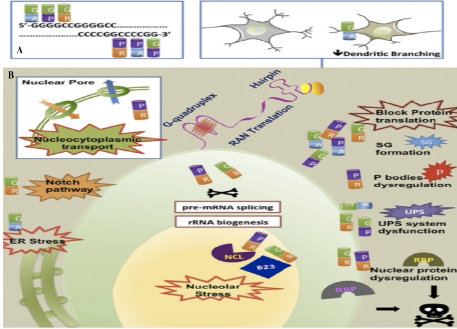
Şekil 2.9. DPR'lerin etkilediği patojenik mekanizmalar (Wen vd., 2017)
