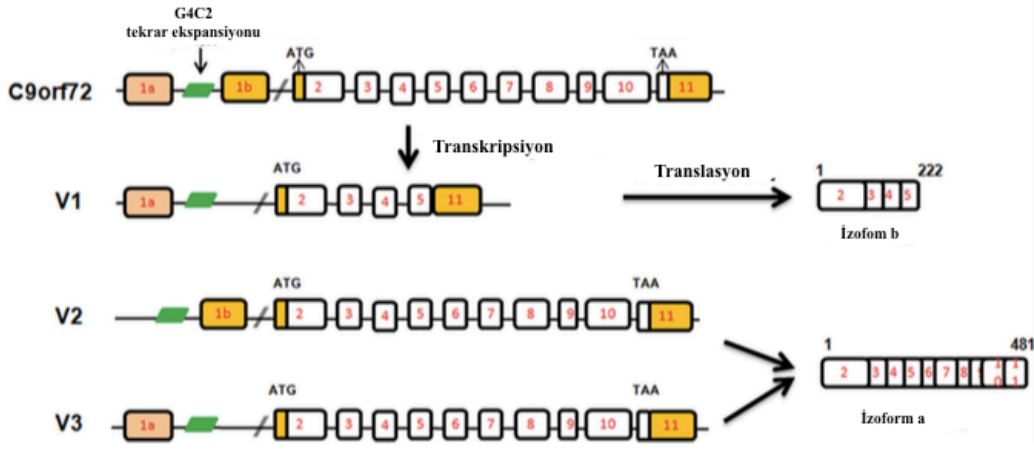
Şekil 2.5. C9orf72 geninin yapısı (Kumar, Islam, Ahmad, & Hassan, 2016)
