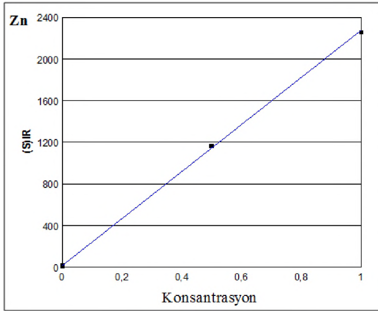
Şekil 7. Çinko eser elementinin kalibrasyon eğrisi.
