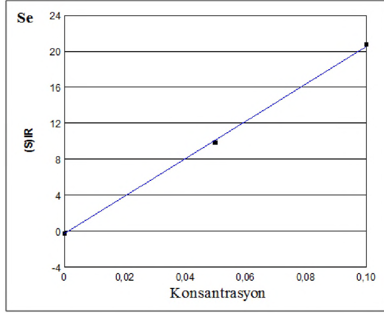
Şekil 8. Selenyum eser elementinin kalibrasyon eğrisi.
