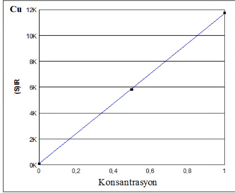
Şekil 4. Bakır eser elementinin kalibrasyon eğrisi
