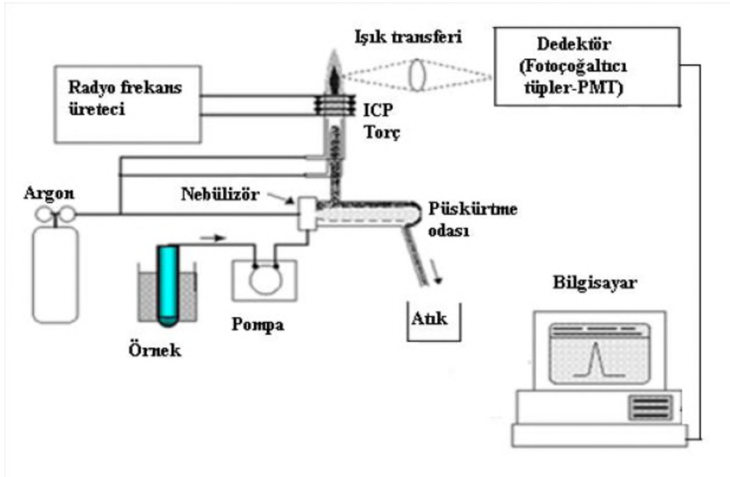
Şekil 3. ICP-OES cihazının çalışma prensibinin şematik görünümü (95).
