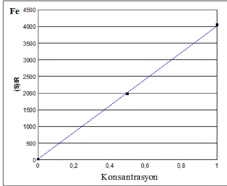
Şekil 5. Demir eser elementinin kalibrasyon eğrisi.
