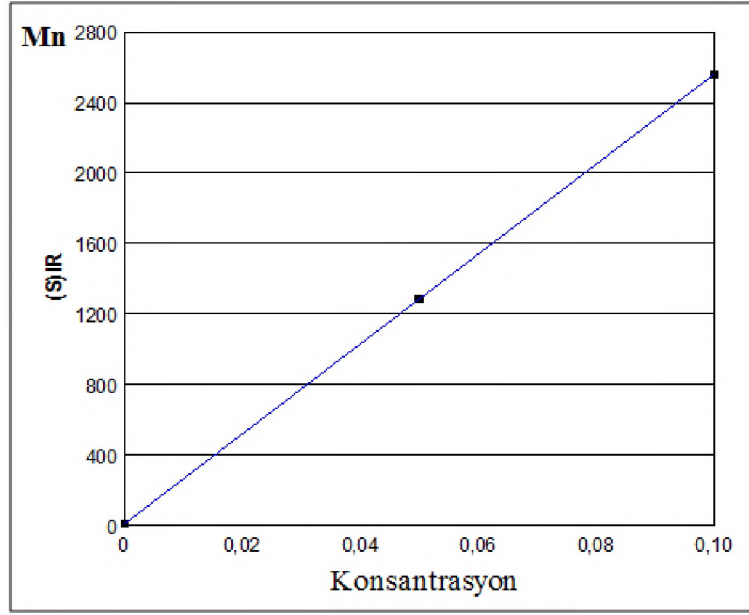
Şekil 6. Mangan eser elementinin kalibrasyon eğrisi.
