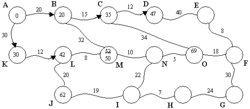
Şekil 2.38 L düğümünden gelen bağlantı M düğümünün önceki değerini iptal eder.
