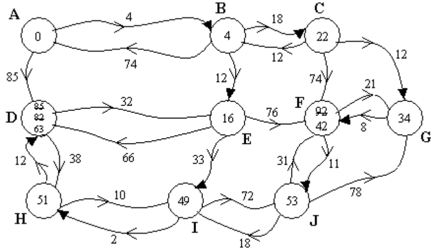
Şekil 2.52 En az dallanan ağaç.
