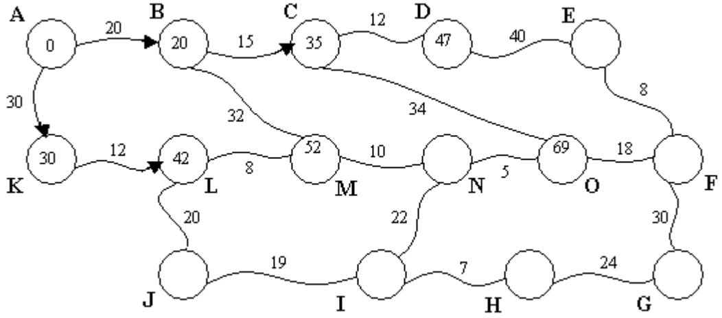
Şekil 2.37 En küçük değer 42 ile L düğümü.
