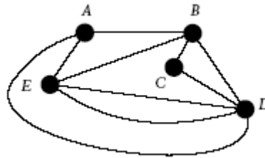
Şekil 2.23 Çoklu graf
