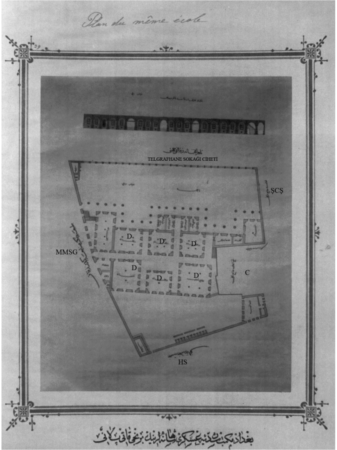
Fotoğraf No 129: Bağdat Mekteb-i Rüşsdiye-i Asker-i Şahanelerinin Birinci Kat Planı
