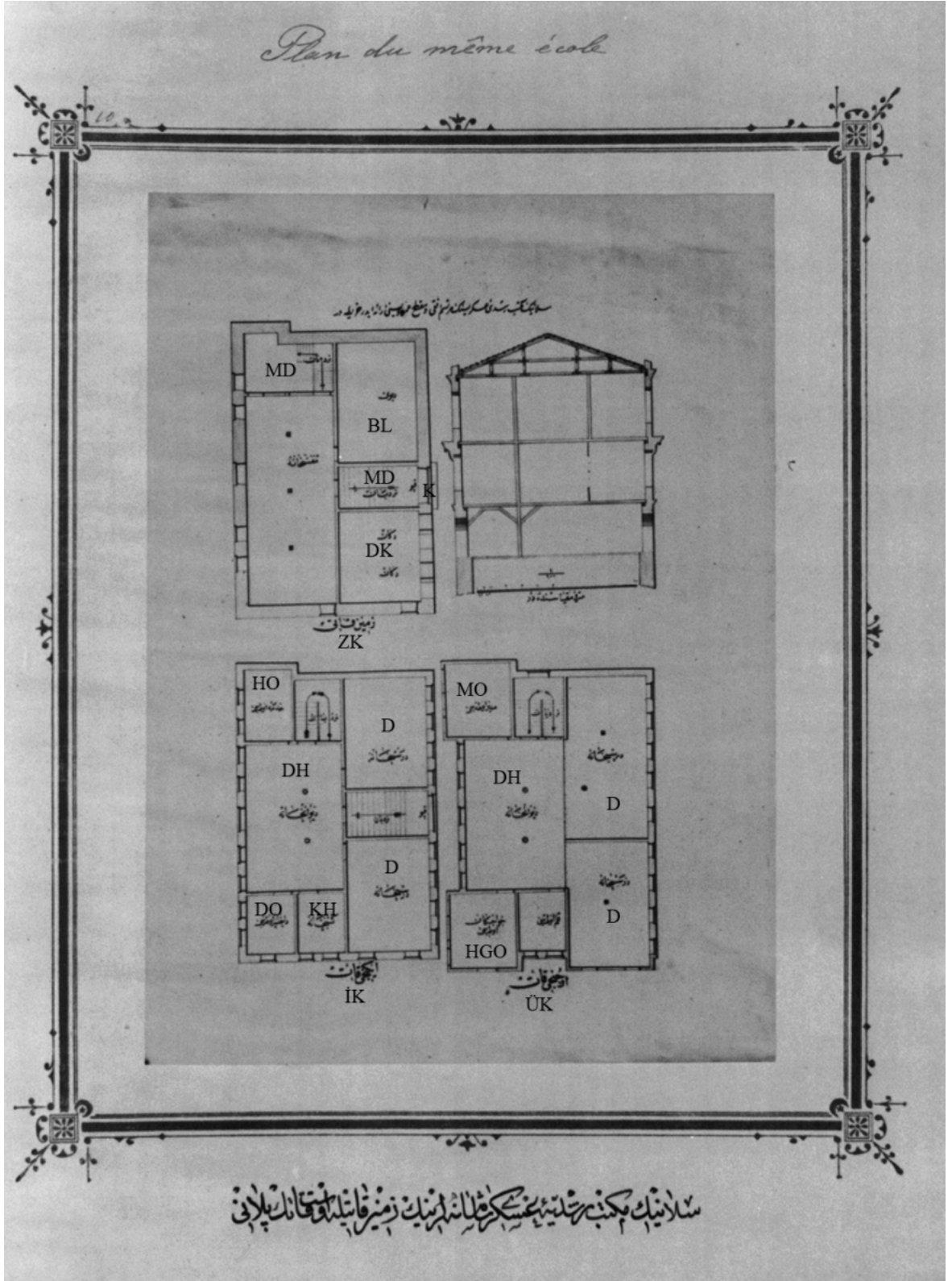
Fotoğraf No 150: Selanik Mekteb-i Rüşdiye-i Askeri Şahaneleri Zemin Katla Üst Katın Planı
