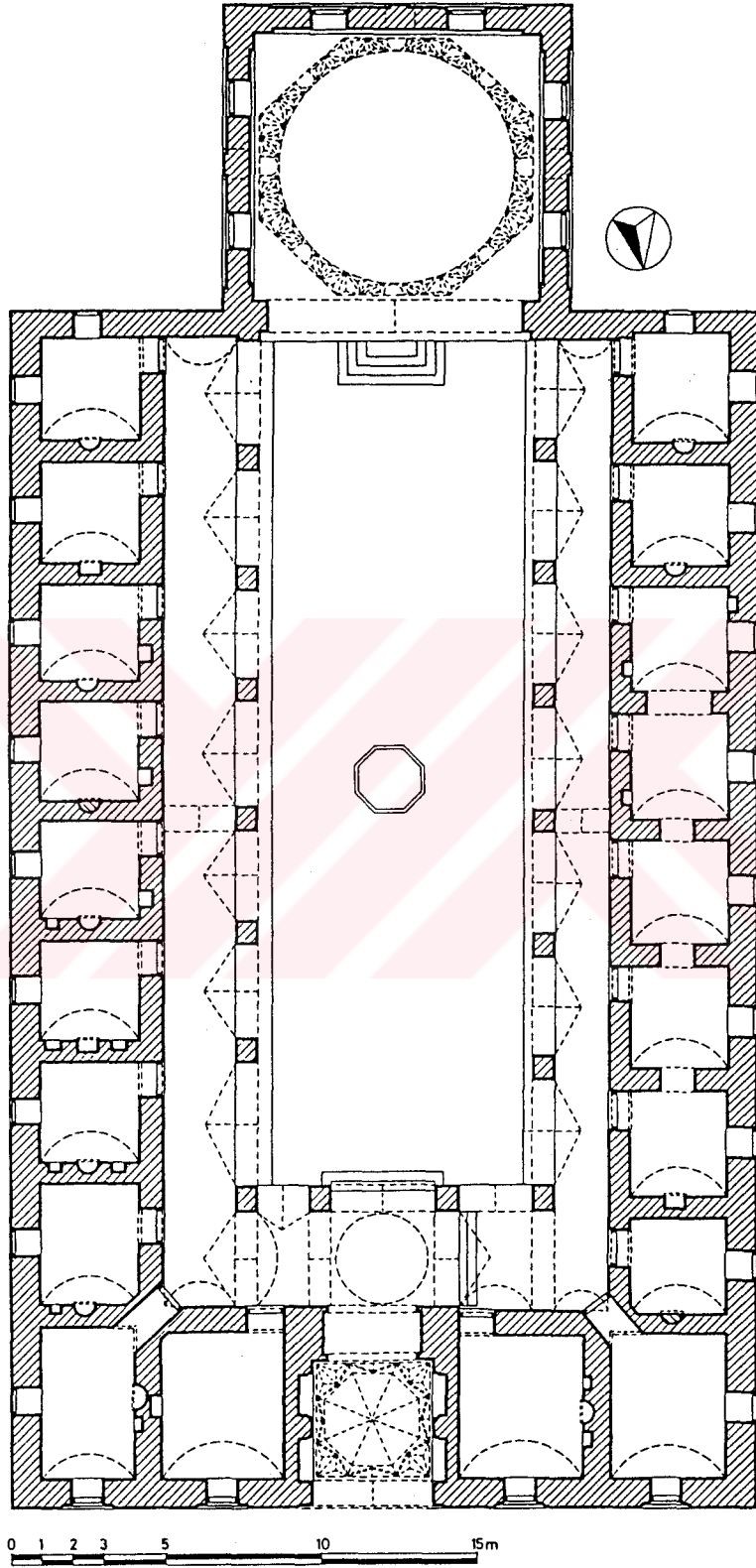
Şekil 9- Bursa Yıldırım Medresesi. Plan. (E.H. Ayverdi'den işlenerek)
