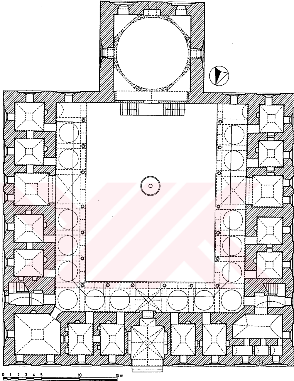
Şekil 38- Bursa Yeşil Medrese. Plan. (E.H. Ayverdi'den işlenerek)
