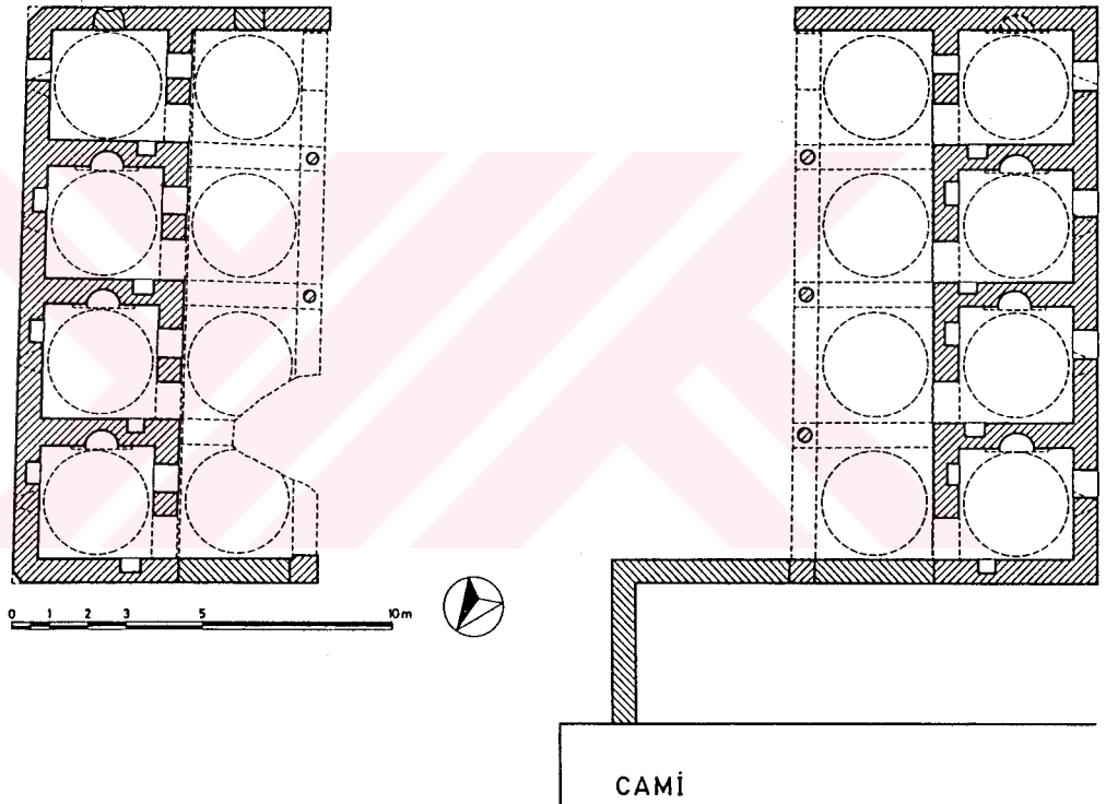
Şekil 77- Bayındır Hacı Sinan Medresesi. Plan.
