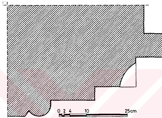
Şekil 21 Bursa Yıldırım Medresesi. Giriş cephesinin doğu kanadında, girişe yakın pencerenin profili
