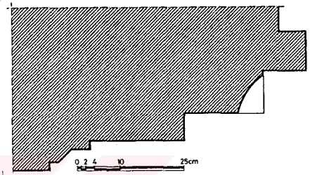
Şekil 18- Bursa Yıldırım Medresesi Giriş cephesinin doğu kana- dında, köşeye yakın pencere- nin profili.
