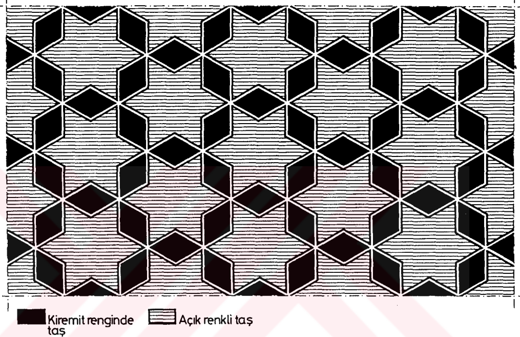
Şekil 8- Bursa Murad Hüdavendigâr Medresesi. Revakın batı cephesinde yer alan süsleme.
