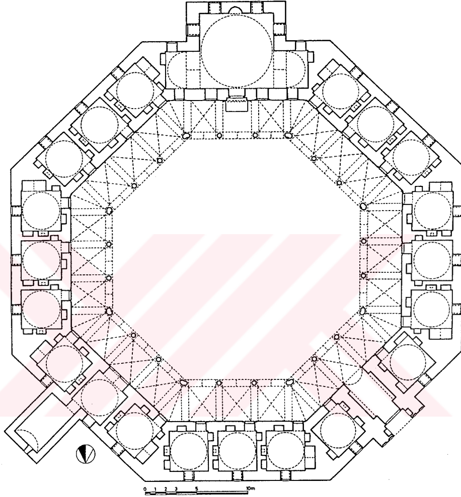
Şekil 74- Amasya Kapağası Medresesi. Plan. (V.G. Müdürlüğü'nden işlenerek)
