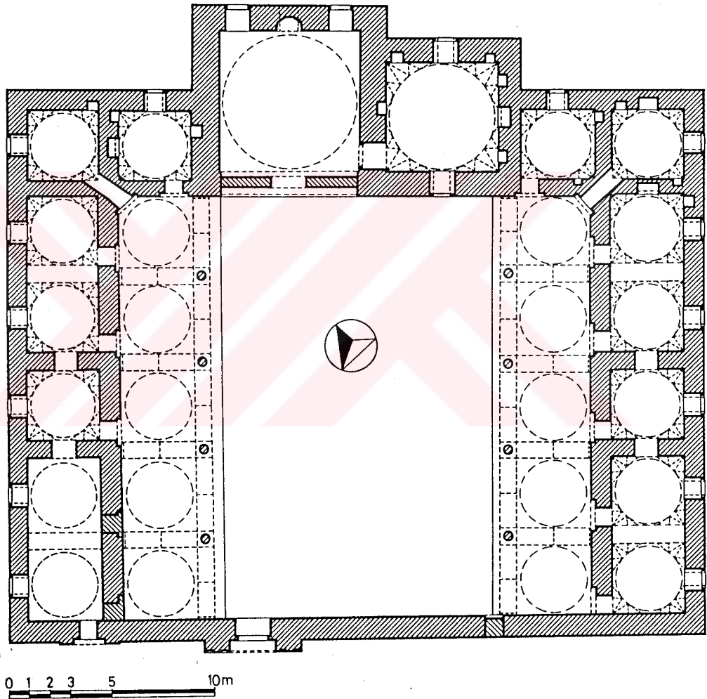
Şekil 56- Afyon Gedik Ahmed Paşa Medresesi. Plan. (E.H.Ayverdi'den işlenerek)
