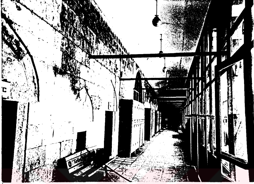
Resim 95- Edirne Peykler Medresesi. Batı revakının içten görünüşü.
