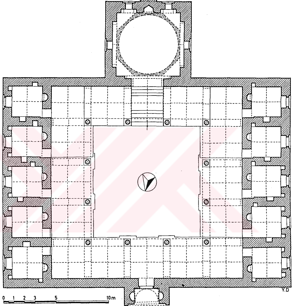
Şekil 48- Manisa Sinan Bey Medresesi. Plan.
