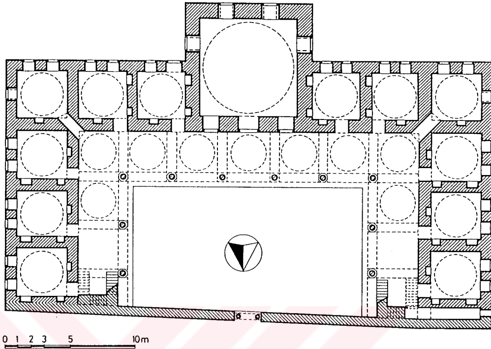
Şekil 79- İstanbul Atik Ali Paşa Medresesi. Rölöve planı.
