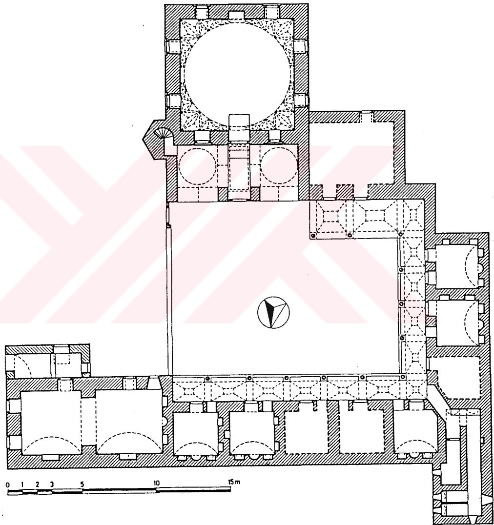
Şekil 75- Amasya Ayas Ağa Medresesi. Plan.
