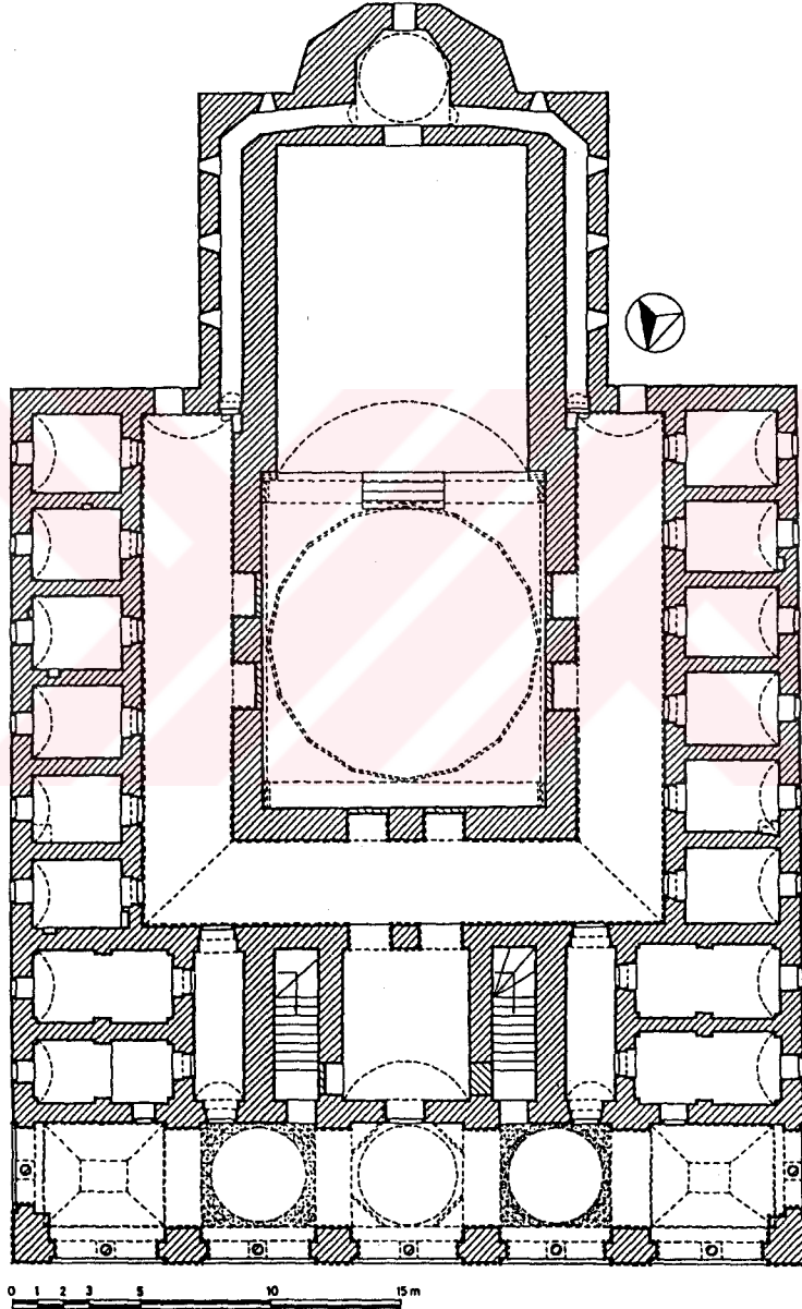
Şekil 4- Bursa Murad Hüdavendigâr Medresesi. Plan. (E.H. Ayverdi'den işlenerek)
