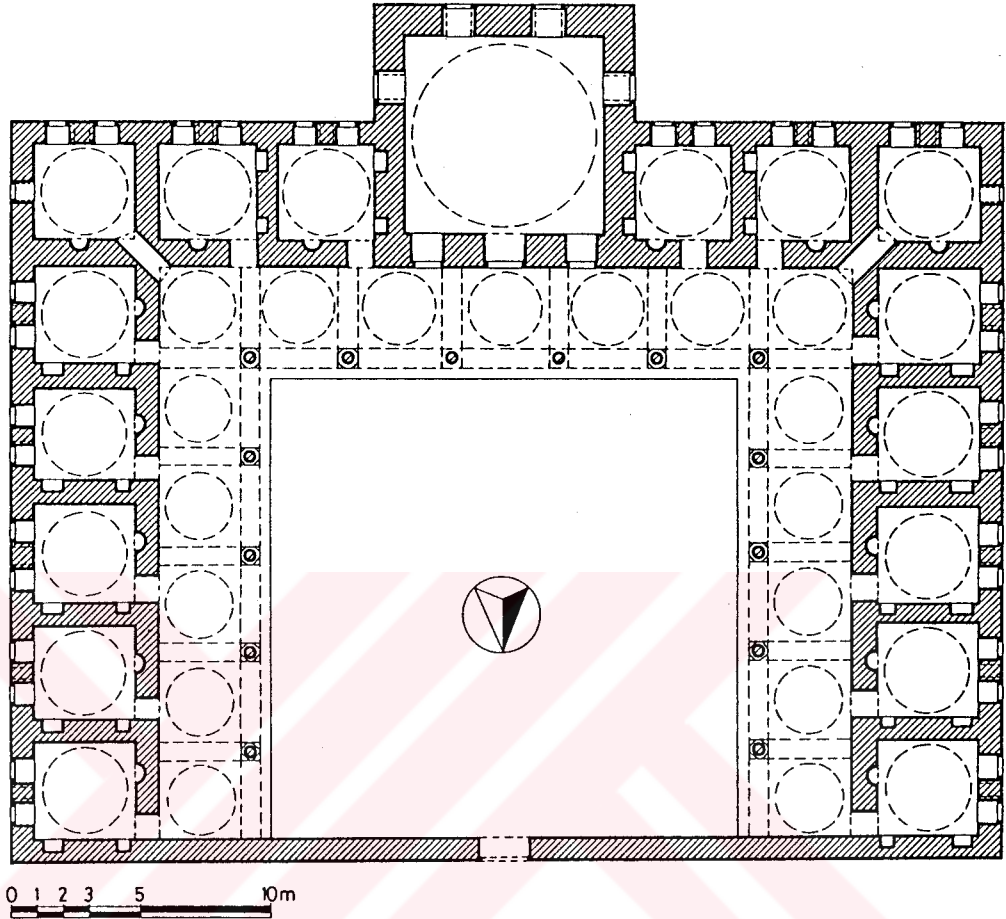
Şekil 78- İstanbul Atik Ali Paşa Medresesi. Restitüsyon planı. (E.H. Ayverdi'den)
