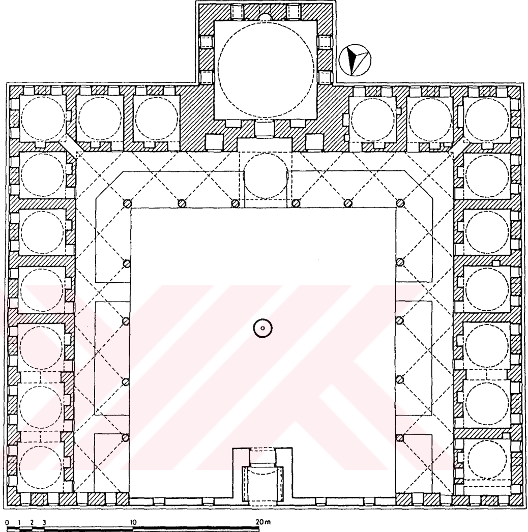
Şekil 66- Amasya II. Bayezid Medresesi. Plan. (E.H. Ayverdi'den işlenerek)
