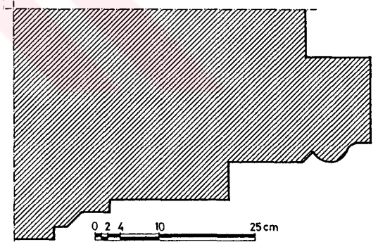
Şekil 20- Bursa Yıldırım Medresesi Giriş cephesinin batı kana- dında, girişe yakın pencere- nin profili.
