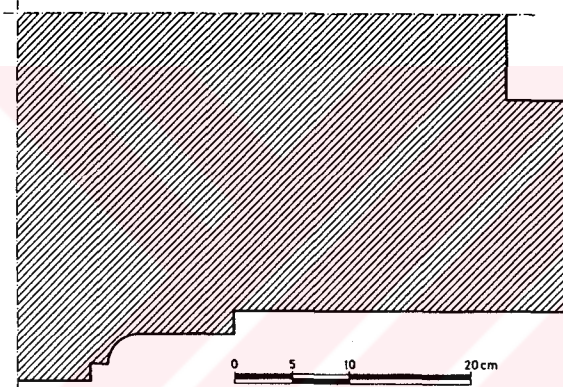
Şekil 35- Merzifon Çelebi Sultan Mehmed Medresesi. Pencere profili.
