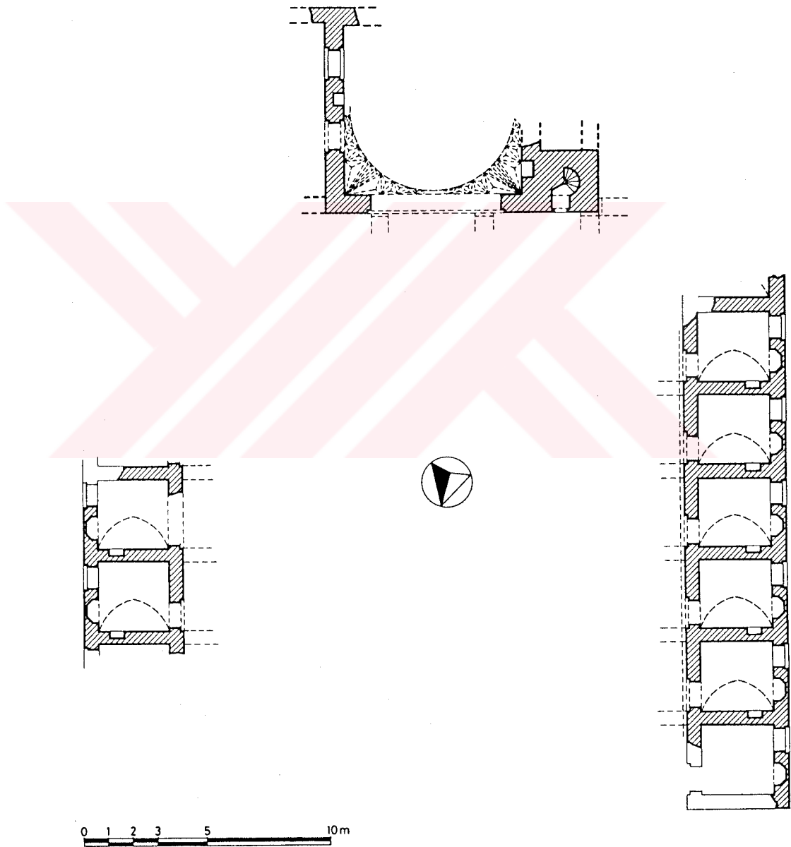
Şekil 58- Tire Molla Arap Medresesi. Plan. (İ. Aslanoğlu'dan işlenerek)
