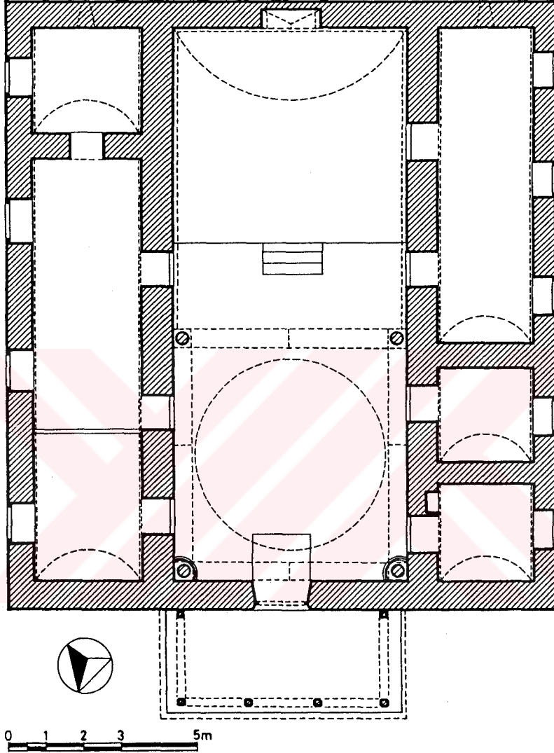
Şekil 2- Bursa Lala Şahin Paşa Medresesi. Plan.
