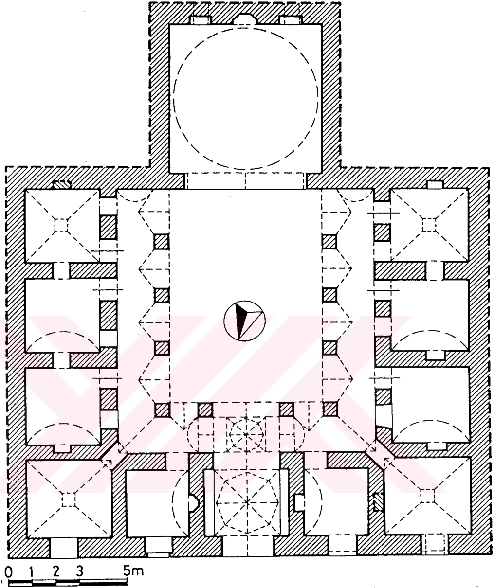
Şekil 82- Bursa Gökdere Medresesi. Plan.
