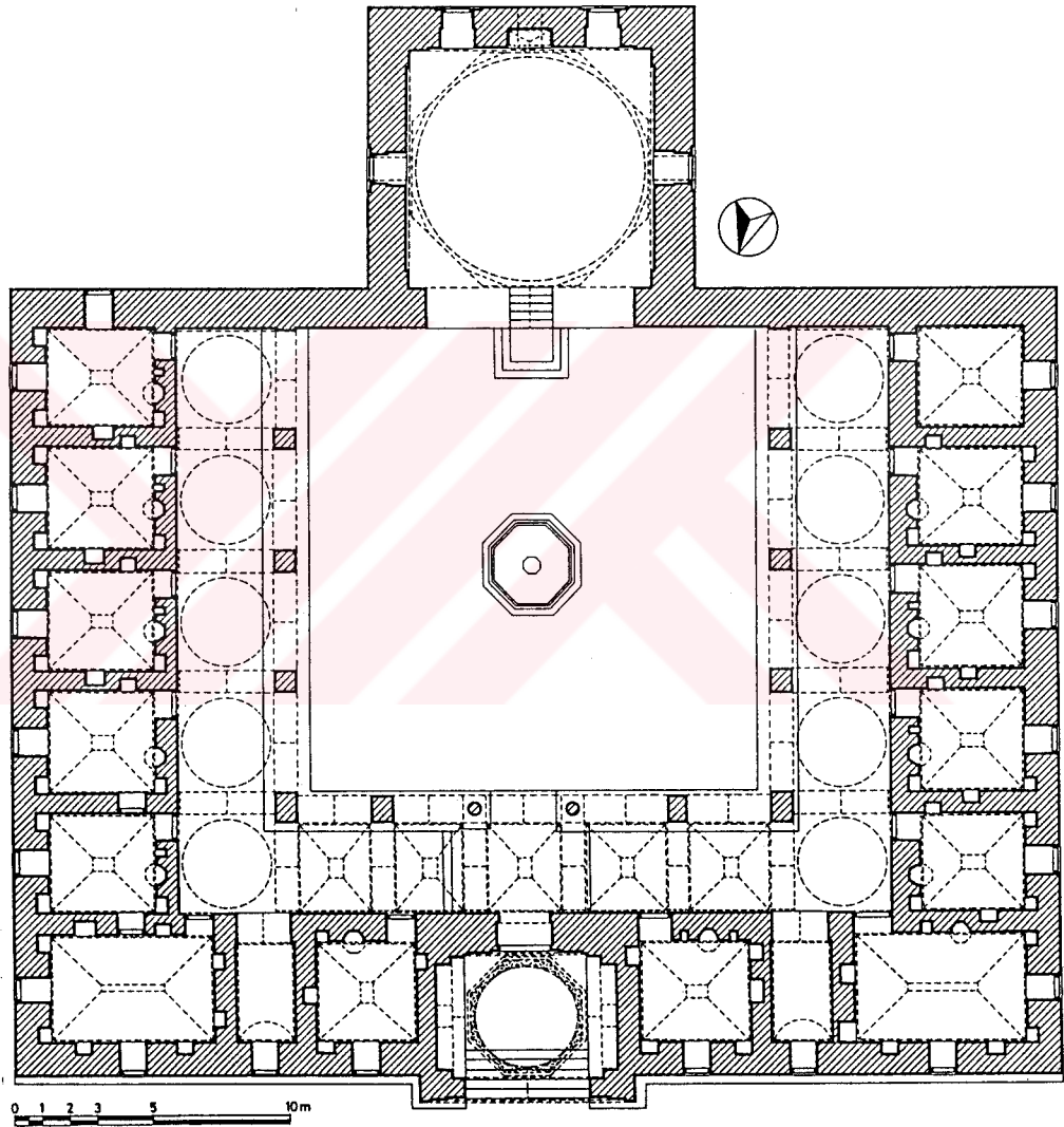
Şekil 42- Bursa Muradiye Medresesi. Plan. (E.H. Ayverdi'den işlenerek)
