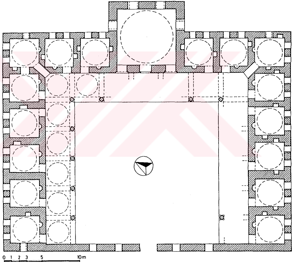
Şekil 65- İstanbul Duvud Paşa Medresesi. Plan. (E.H. Ayverdi'den işlenerek)
