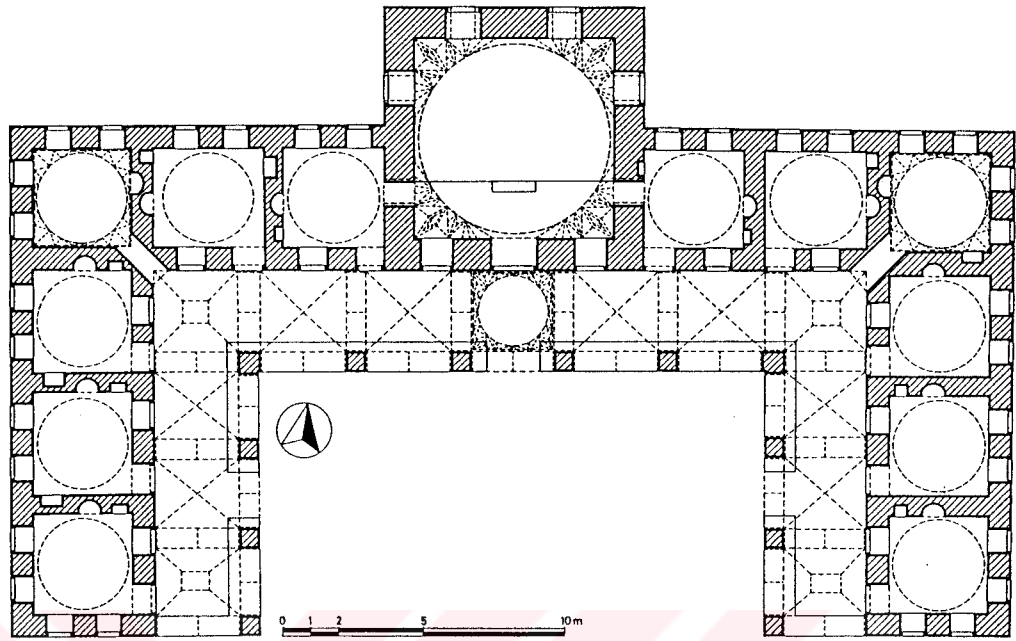
Şekil 63- İnegöl İshak Paşa Medresesi. Plan. (E.H. Ayverdi'den işlenerek)
