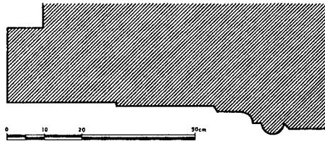
Şekil 70- Edirne II. Bayezid Medresesi. Pencere profili.
