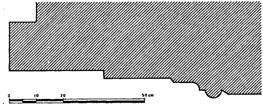
Şekil 71- Edirne II. Bayezid Medresesi. Taçkapı profili.
