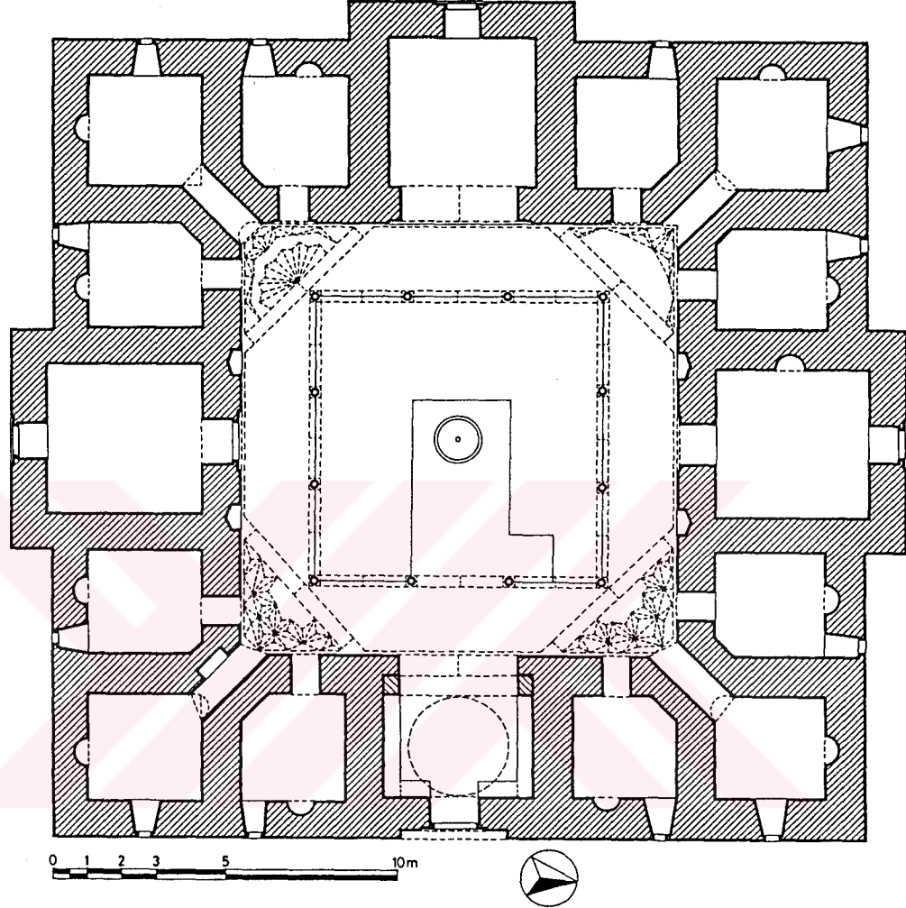
Şekil 28- Gümüş Hacı Halil Paşa Medresesi. Plan. (E.H. Ayverdi'den işlenerek)
