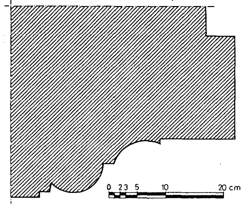
Şekil 30- Gümüş Hacı Halil Paşa Medresesi. Kuzey ve batı kanadındaki dersanelerin pencere profilleri.
