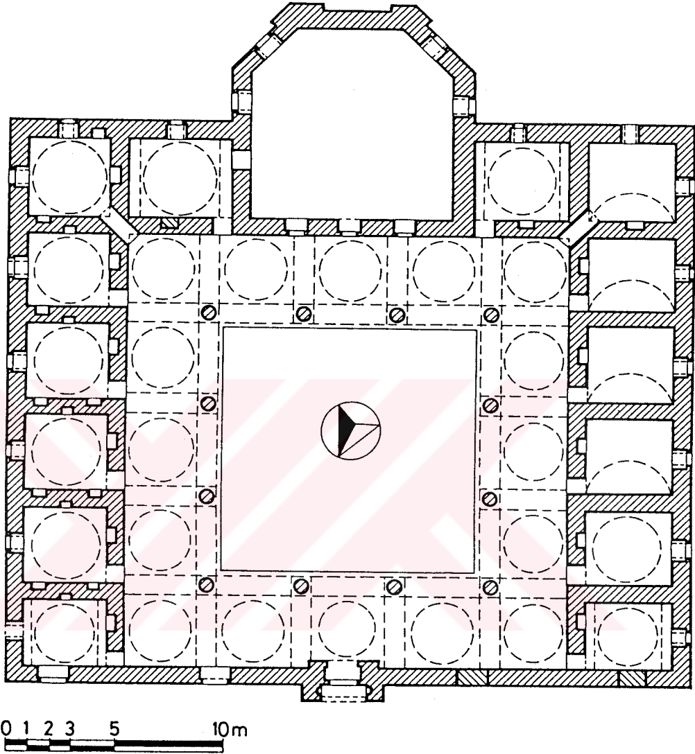
Şekil 67- İstanbul Koca Mustafa Paşa Medresesi. Plan. (E.H. Ayverdi'den işlenerek)
