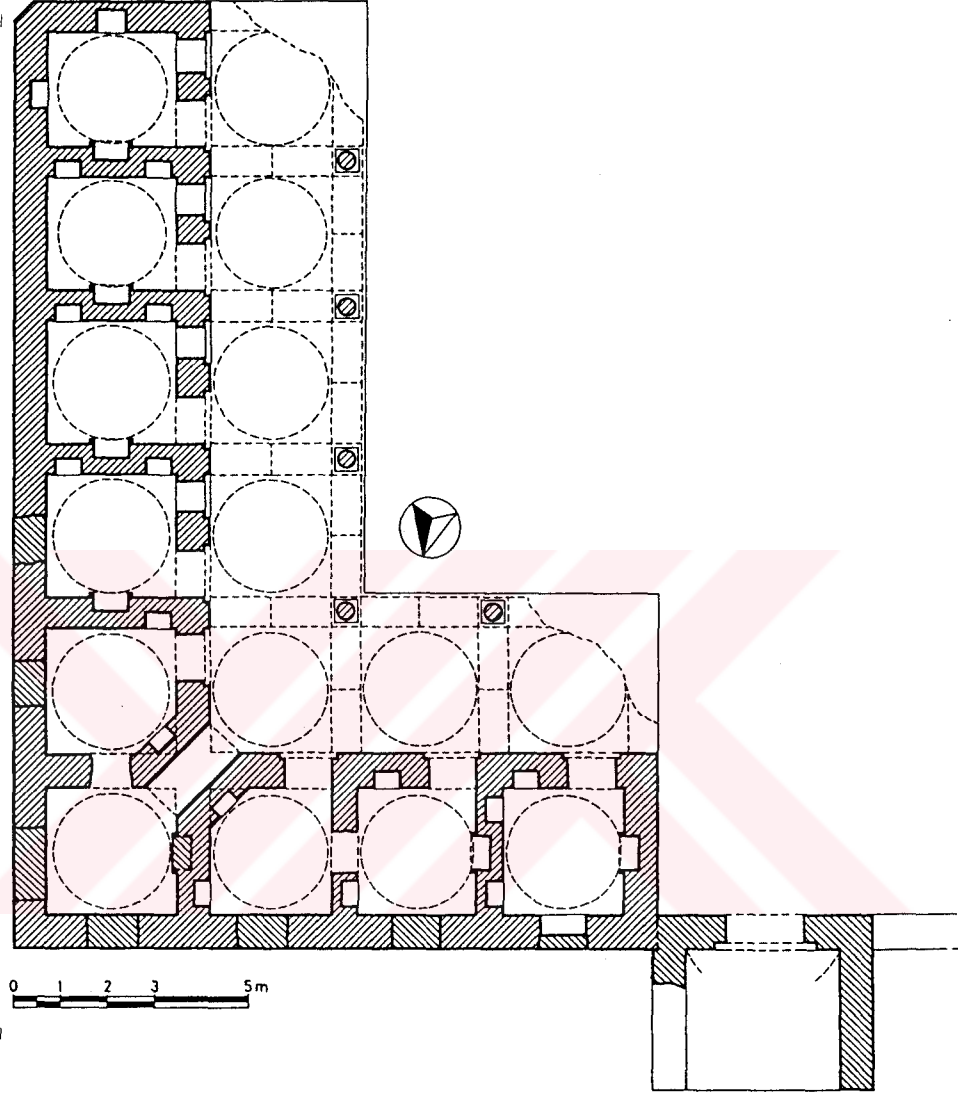
Şekil 81- Hereke (Düzce) Köyü Medresesi. Plan.
