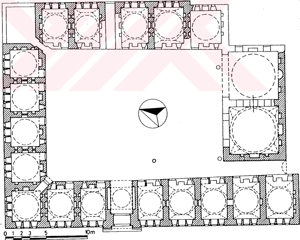
Şekil 47- Edirne Saatli Medrese. Plan.
