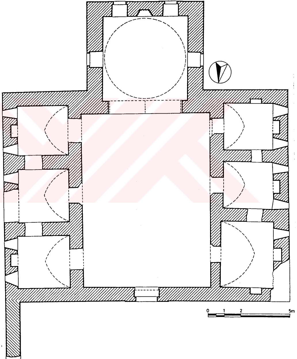
Şekil 50- Yolpınar Köyü Kasım Bey Medresesi. Plan.
