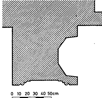
Şekil 68- İstanbul Koca Mustafa Paşa Medresesi. Taçkapı profili.
