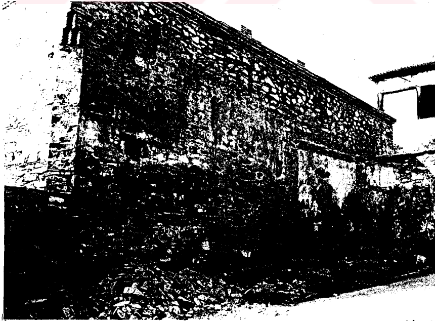
Resim 134- Bayındır Hacı Sinan Medresesi. Batı cephesinin onarımdan sonraki durumu. (Kasım 1996)
