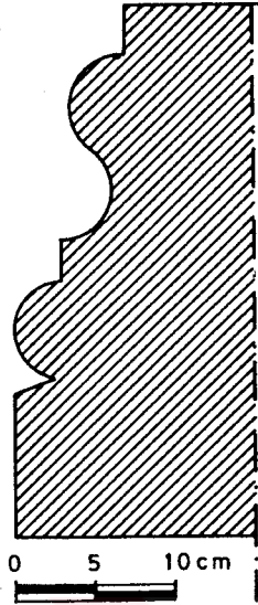
Şekil 72-Edime II. Bayezid Medresesi. Sütun kaidesi profili.
