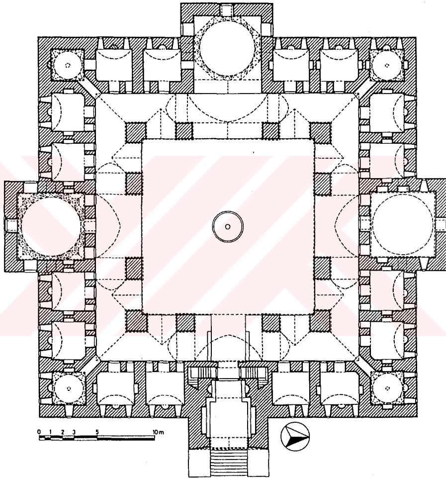
Şekil 34- Merzifon Çelebi Sultan Mehmed Medresesi. Plan. (E.H. Ayverdi'den işlenerek)
