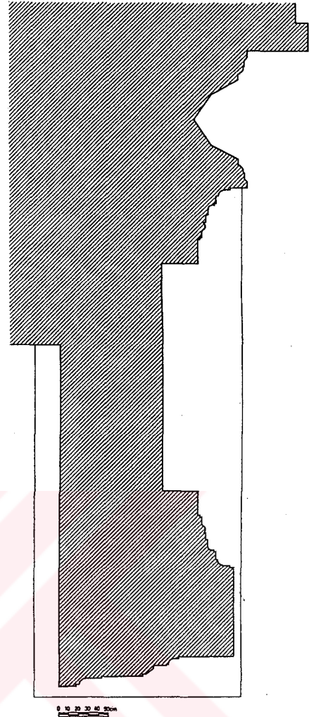
Şekil 36- Merzifon Çelebi Sultan Mehmed Medresesi. Taçkapı profili.
