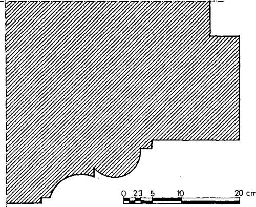
Şekil 29- Gümüş Hacı Halil Paşa Medresesi. Kuzey ve batı kanadındaki dersanelerin pencere profilleri.
