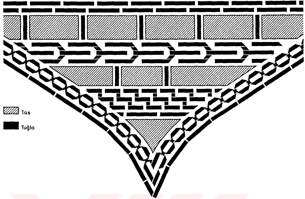
Şekil 27- Bursa Subaşı Eyne Bey Medresesi. Revak cephesinin kemer köşeliklerinde yer alan süsleme
