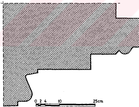
Şekil 19- Bursa Yıldırım Medresesi. Giriş cephesinin doğu kana- dında, girişe yakın pencere- nin profili.
