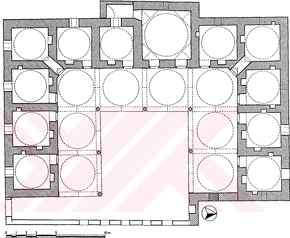
Şekil 1- İznik Süleyman Paşa Medresesi. Plan.
