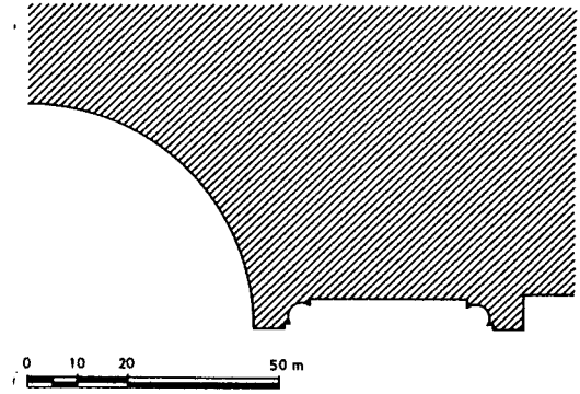
Şekil 73-Edime II. Bayezid Medresesi. Ocak profili.
