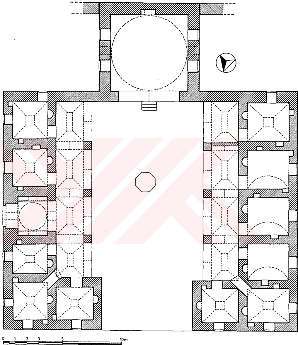
Şekil 57- Bursa Ahmed Paşa Medresesi. Plan. (E.H. Ayverdi'den işlenerek)
