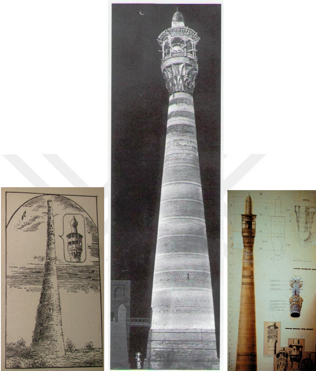
Kutluğ Timur minaresinin külâhı ve aleminin tahmin edilmekte olan şekli. 1318
