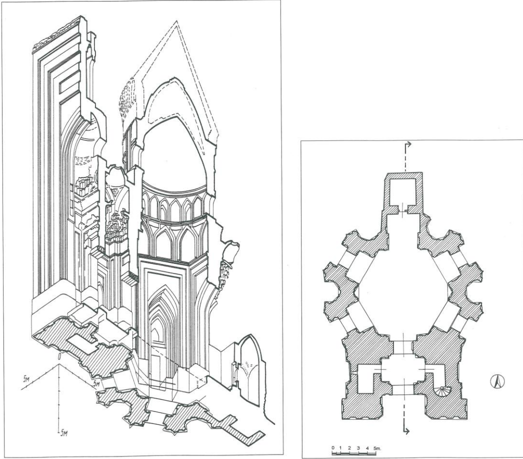
Törebek Hanım Türbesi aksonometrik kesit ve planı. 1321
