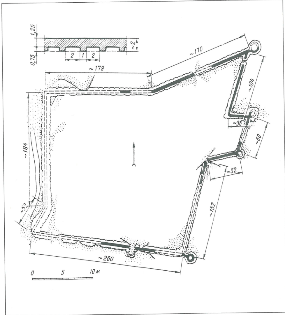
Gürgenç'te şehrin içkalesi olduğu tahmin edilen Ak-kale'nin planı. 1325
