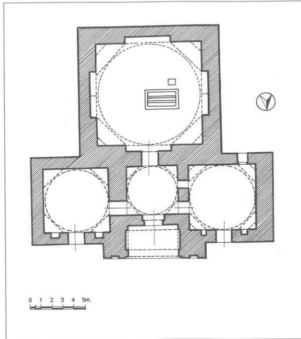
Necmeddîn-i Kübra Türbesi planı. 1322
