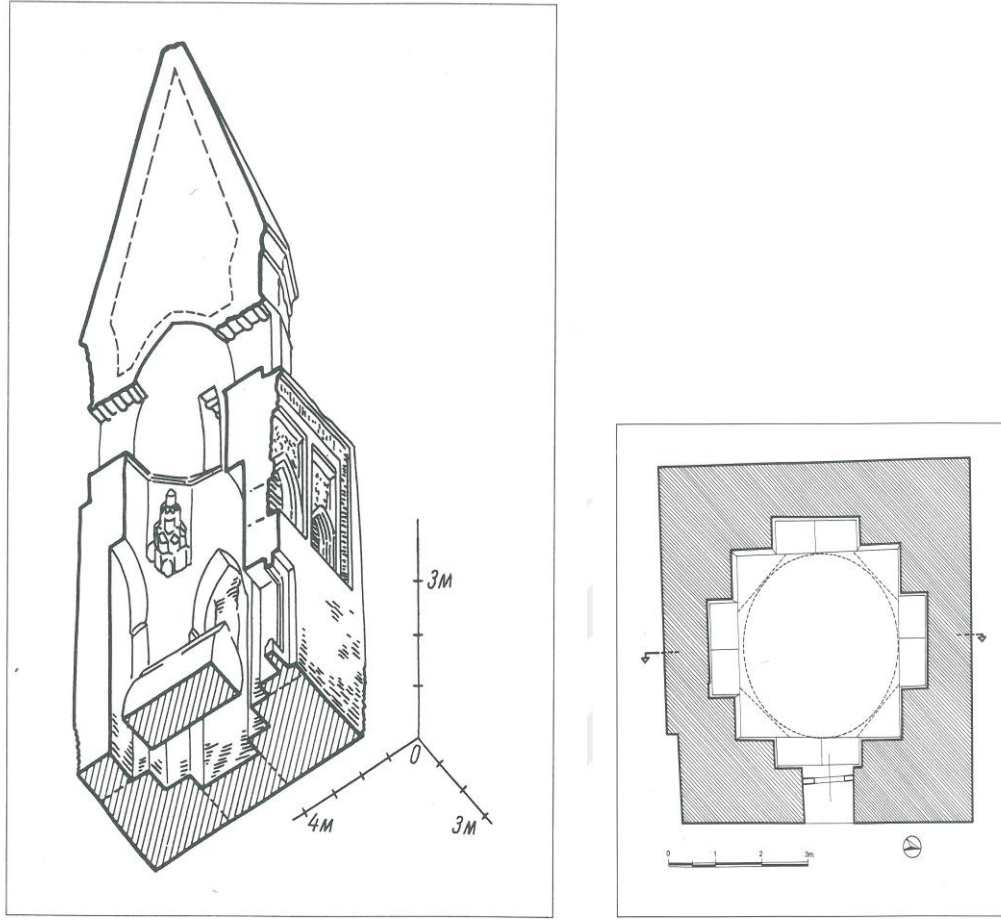
Fahreddin er-Râzî veya İl Arslan Türbesi aksonometrik kesit ve planı. 1319
