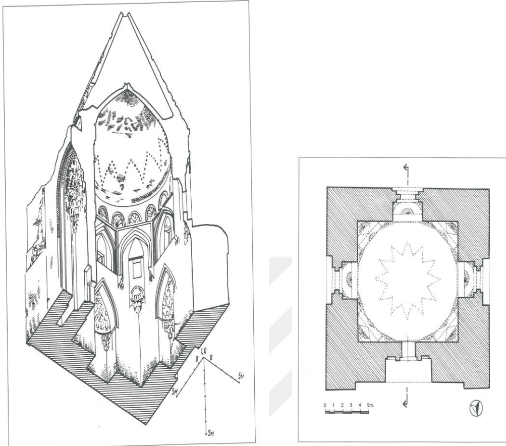
Sultan Tekiş Türbesi aksonometrik kesit ve planı. 1320
