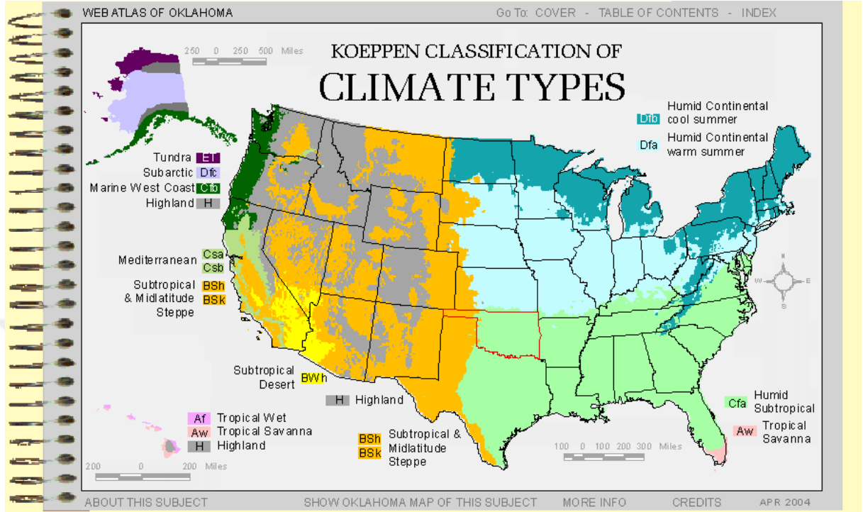
Figür 3: Koeppen İklim Çeşitleri Sınıflandırmasına göre ABD’de bölgelere göre iklim çeşitleri Bu iklim çeşitliliğine bağlı olarak ülkede yirmi beş bine yakın bitki türü ve binden fazla ağaç türü vardır. Ulusal parkları ise şehirler kadar geniş yer kaplar.
