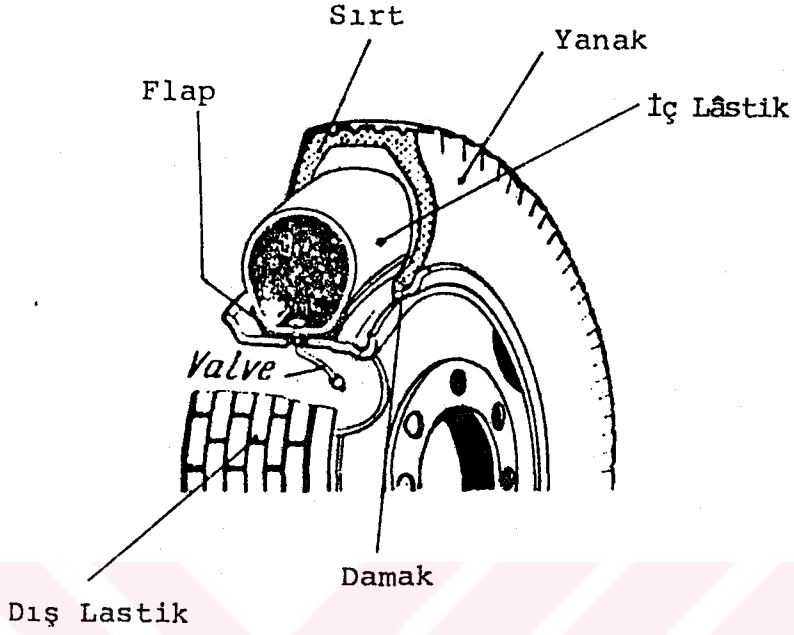
Çizim 5-1 : Oto Lastiği Ana Parçaları
