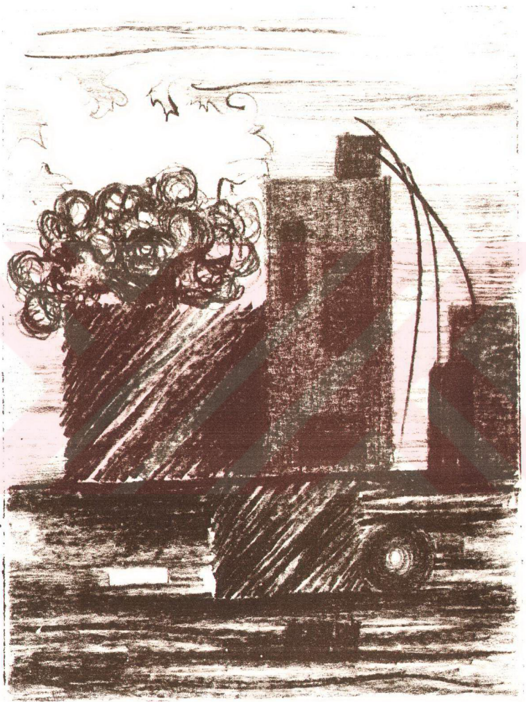
BASKI 11 - T.E.Griffits Yöntemi
