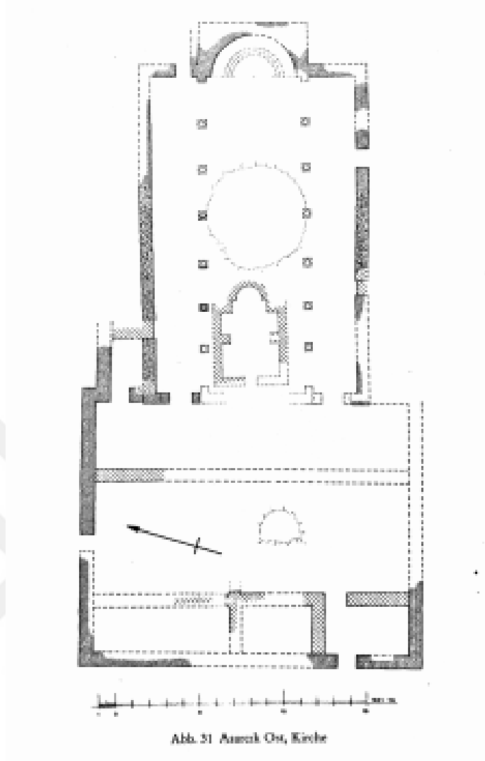
Çizim 20. Asarcık Doğu Kilisesi
