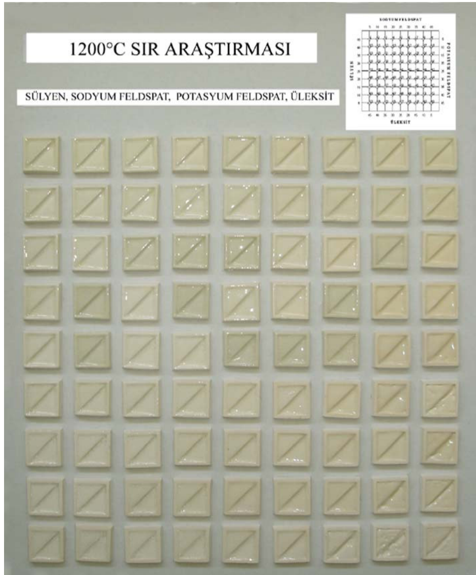
Resim 53. 1200°C Sıcaklıkta Gelişebilen Bakır Kırmızısı Sır Araştırmasında Kullanılan Farklı Sır Hammadde Karışım Çizelgesi Pişirim Sonuçları
