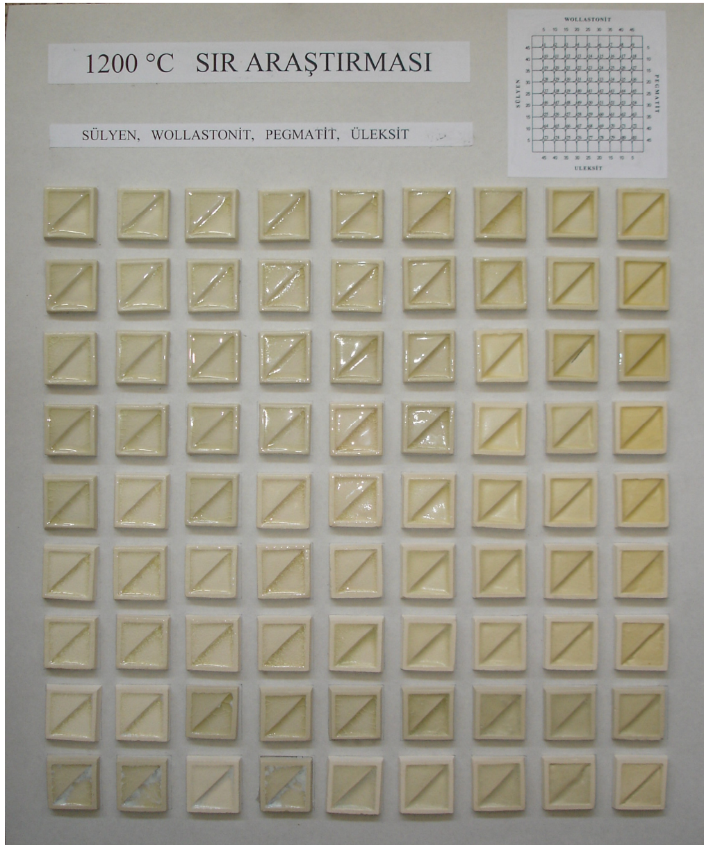
Resim 54. 1200°C Sıcaklıkta Gelişebilen Bakır Kırmızısı Sır Araştırmasında Kullanılan Farklı Sır Hammadde Karışım Çizelgesi Pişirim Sonuçları
