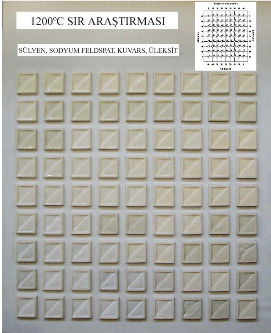
Resim 47. 1200°C Sıcaklıkta Gelişebilen Bakır Kırmızısı Sir Araştırmasında Kullanılan Farklı Sir Hammadde Karışımları Çizelgesi Pişirim Sonuçları
