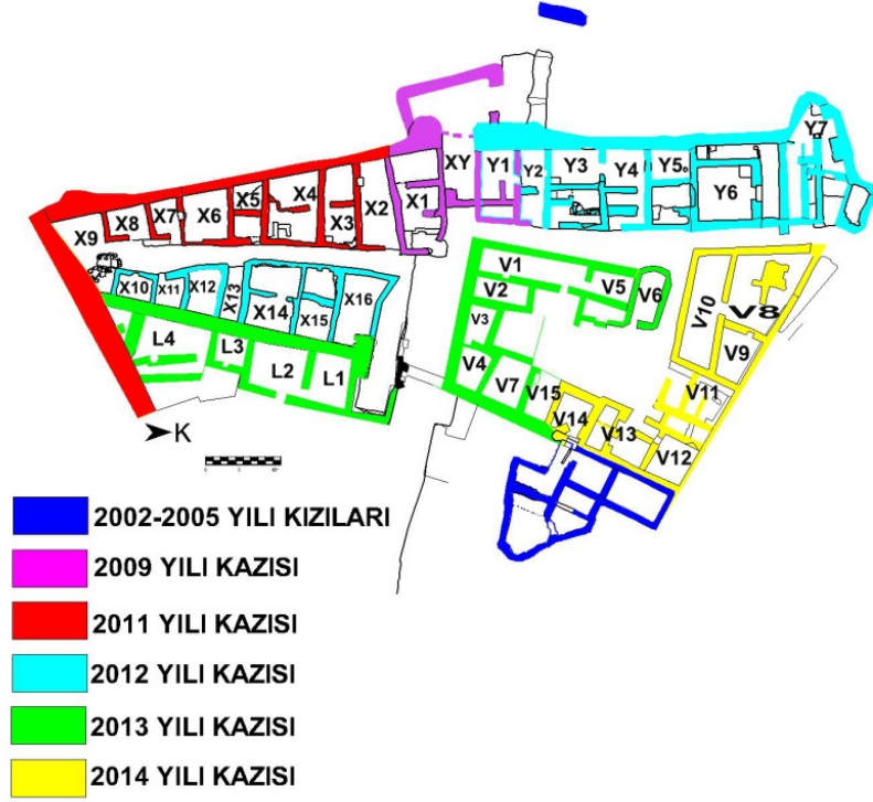
Çizim 1. Karacahisar Kalesi Giriş Bölümü Planı (Ali Gerengi)
