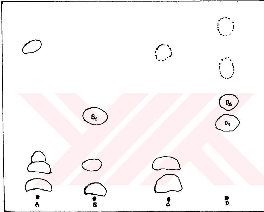
Şekil 4.3. İnce tabaka kromatogramı. R_f değeri 0.5 dolaylarında olan ekstreye ait lekenin ( D_1 ), kontrol grubu (C) ve 250 mg/kg Hyp grubu (A) sıçanların safralarına ait kromatogramlarda bulunmadığı, fakat sıçanların 500 mg/kg Hyp grubunda bulunduğu ( B_1 )görülmektedir.
