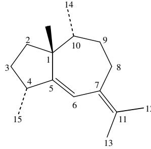
Gaya-5,7(11)-dien (1)
