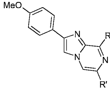
Şema 24. 2-(4-Metoksifenil)imidazo[1,2-a]pirazin
