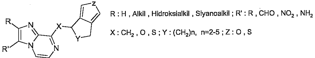
Şema 35. 2,3-Disübstitüe-8-heteroarilimidazo[1,2-a]pirazin
