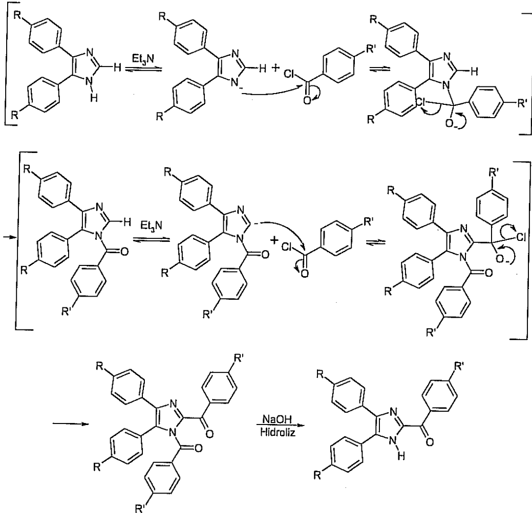
Şema 75. 2-Ariloil-4,5-diarilimidazolün Sentez Mekanizması
