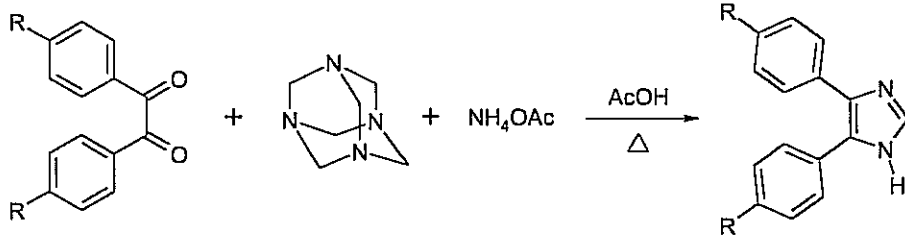
Şema 72. 4,5-Diarilimidazol
