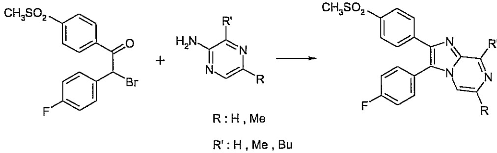
Şema 31. 2,3-Diaril-6,8-disüstitüe İmidazo[1,2-a]pirazin
