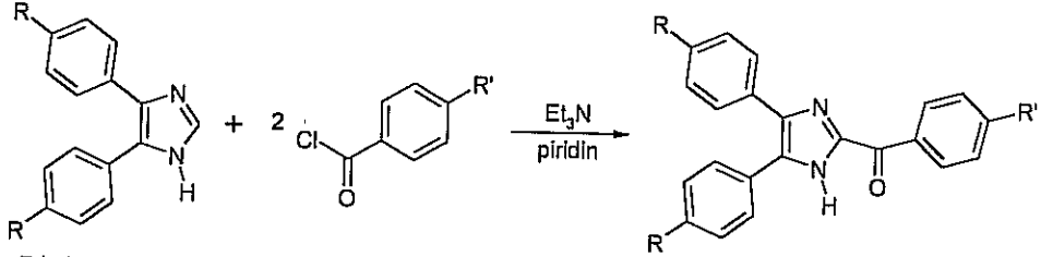
Şema 74. 2-Ariloil-4,5-diarilimidazol
