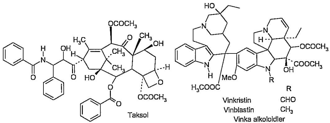
Şema 10. Bazı Kromatin Fonksiyon İnhibitörleri
