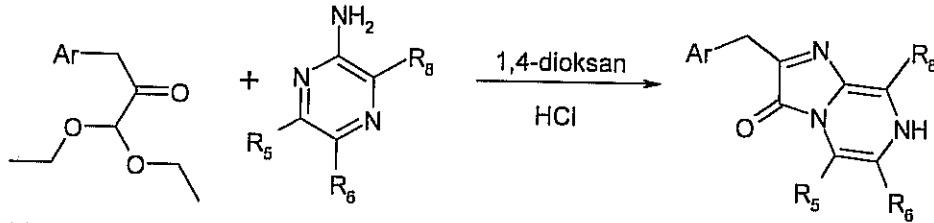
Şema 14. 3,7-Dihidroimidazo[1,2-a]pirazin-3-on
