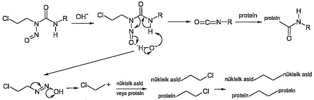
Şema 5. Bazı Nitrozoüreler
