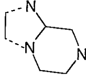
Şema 12. İmidazo[1,2-a]pirazinin 1,2- ve 3,4- Bağ Oluşumu
