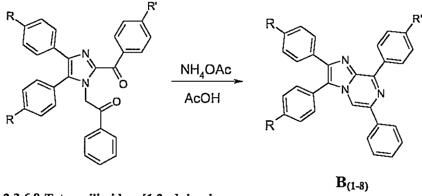
Şema 78. 2,3,6,8-Tetraarilimidazo[1,2-a]pirazin
