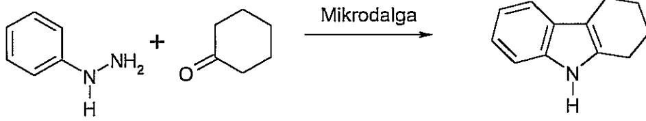
Şema 56. Tetrahidrokarbazol
