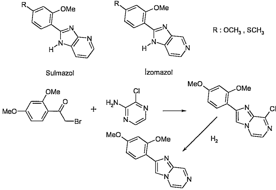
Şema 25. 2-Arylimidazo[1,2-a]pirazin
