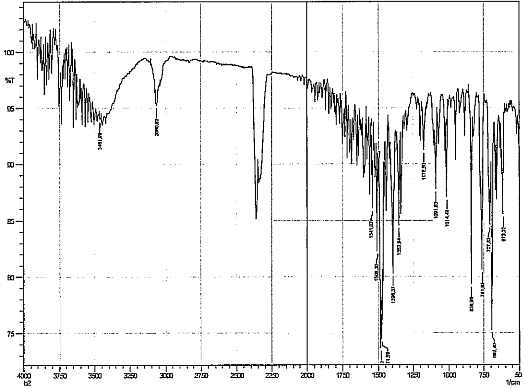
Ek.1.10 Bileşik B 2 'ye ait IR Spektrumu
