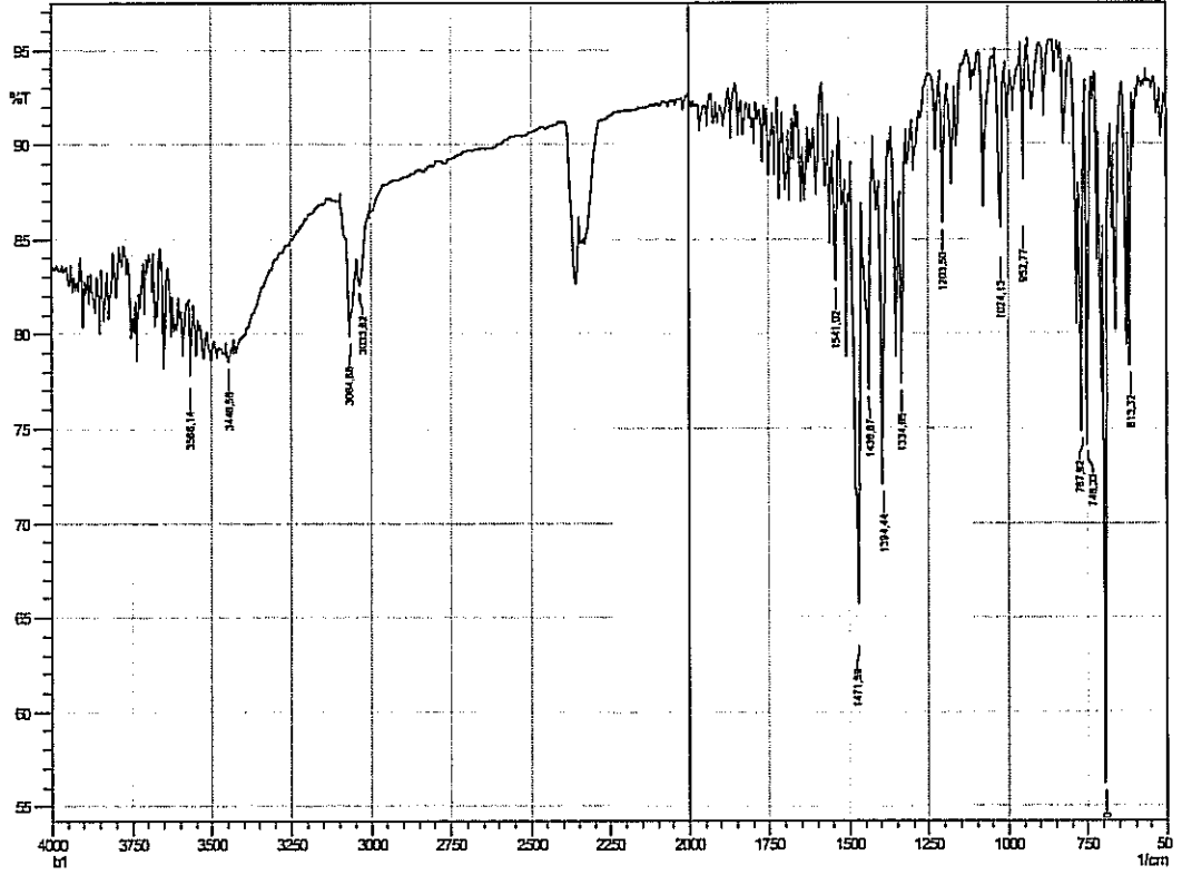
Ek.1.9 Bileşik B 1 'e ait IR Spektrumu
