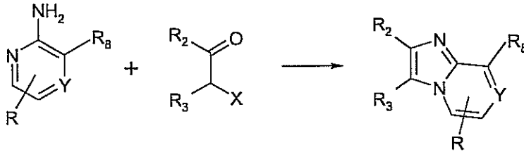
X = Br , Cl ; Y = CH , CCH 3 , CPhCHCH 2 , N ; R = H , CH 3 , CH 2 CH 2 Ph ; R 2 = H , CH 3 R 3 = H , CH 2 CN , OCH 3 , SCH 3 , CH 3 ; R 8 = H , Cl , CHO , PhCH 2 O , PhCH 2 NH , PhCH 2 CH 2 Şema 34. İmidazo[1,2-a]pirazin ve İmidazo[1,2-a]piridin
