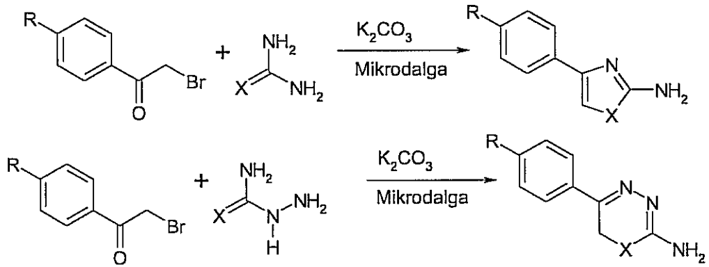
Şema 55. Okzadiazin ve Tiyadiazin Türevleri
