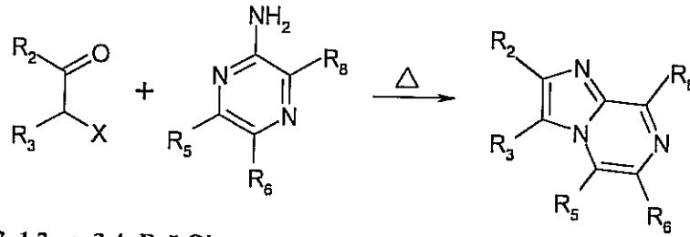
Şema 13. 1,2- ve 3,4- Bağ Oluşumu
