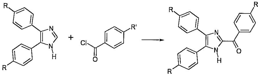
Şema 64. Yöntem E İçin Tahmin Edilen Genel Sentez Şeması
