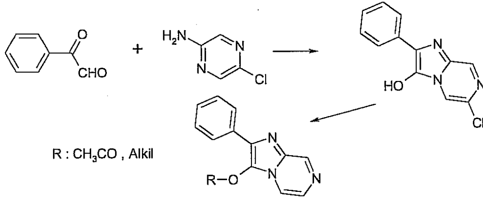
Şema 28. 2,3-Disübstitüe İmidazo[1,2-a]pirazin
