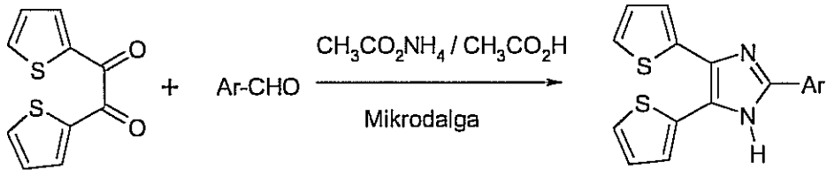
Şema 58. Bazı Ditiyenilimidazol Türevleri
