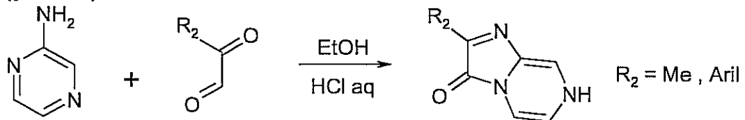
Şema 46. Bazı İmidazo[1,2-a]pirazin-3-on Türevlerinin Sentezi
