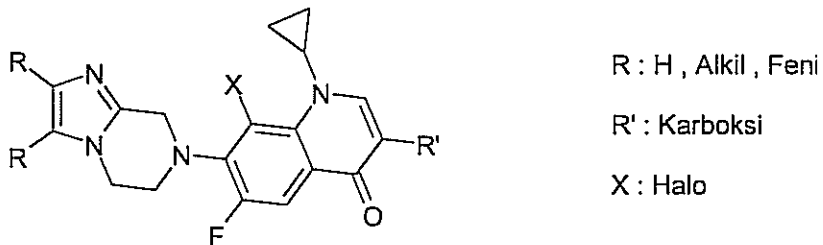
Şema 44. 2,3-Disübstitüe-7-heteroarilimidazopirazin
