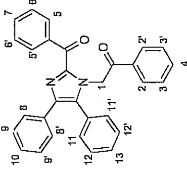
Çizelge 2. 1-(2-Fenil-2-okzoetil)-2-arilolil-4,5-diarilimidazol (A) Türevlerinin 1 H-NMR Spektrum Verileri
