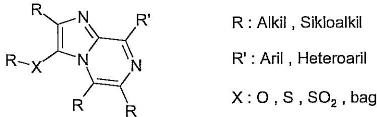
Şema 29. 2,3,5,6,8-Pentasübstitüe İmidazo[1,2-a]pirazin
