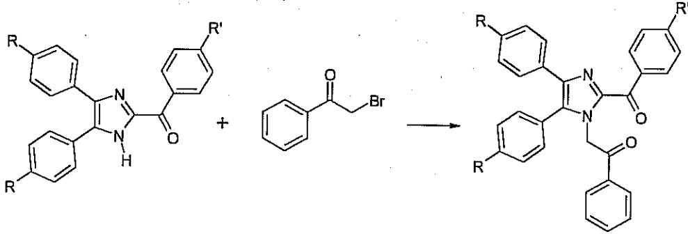
Şema 65. Yöntem F İçin Tahmin Edilen Genel Sentez Şeması
