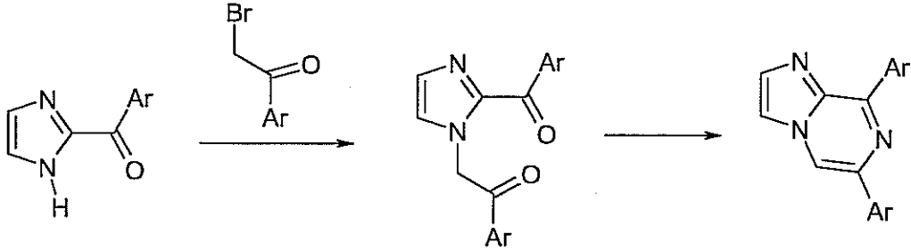
Şema 19. 6,8-Diarilimidazo[1,2-a]pirazin
